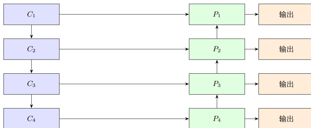
图 32: FPN 结构: 自上而下路径与横向连接
