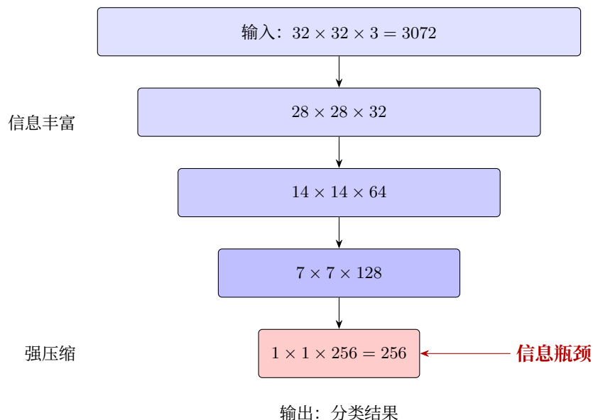
图 28: 信息漏斗：容量瓶颈
