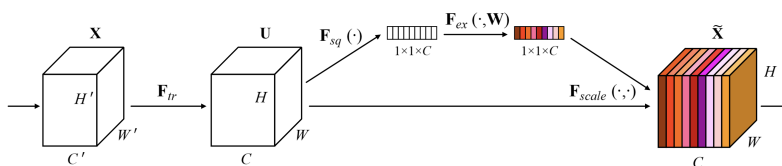
图 20: SE-Net 模块结构: Squeeze \rightarrow Excite \rightarrow Scale
