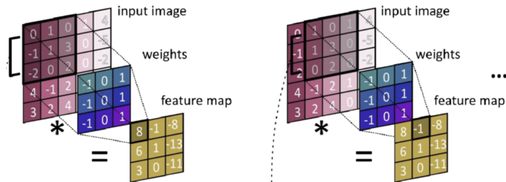
图 5: 参数共享机制示意图
