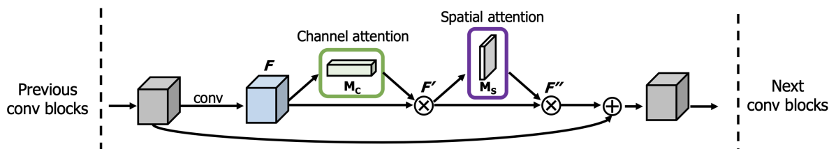
图 24: CBAM-ResNet: 在残差块中插入 CBAM 模块
