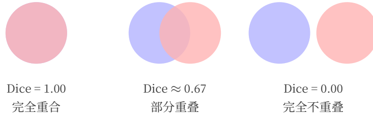
图 4: Dice 系数的可视化
