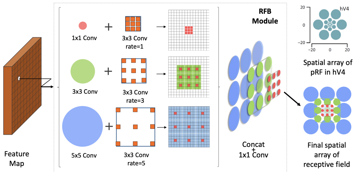
图 10: RFB 模块结构: 三个分支并行, 分别使用不同大小的初始卷积 ( 1 \times 1 、 3 \times 3 、 5 \times 5 ) 配合不同空洞率的 3 \times 3 卷积 (rate=1、3、5), 最后拼接并通过 1 \times 1 卷积融合, 形成多尺度感受野。图片来自 RFB Net 论文。
