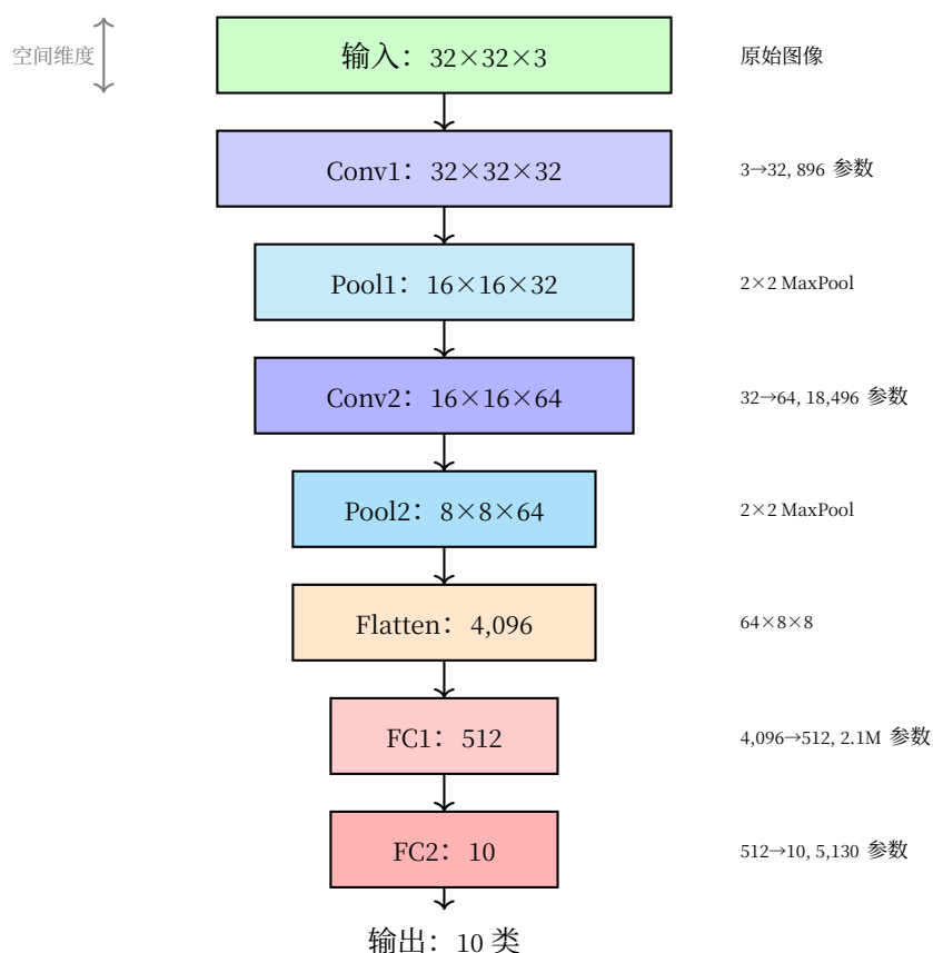
图 15: 基线 CNN 架构：数据流与参数量
