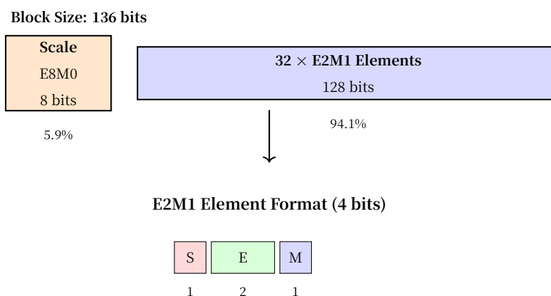
图 2: MXFP4 块结构：32 元素共享一个缩放因子
