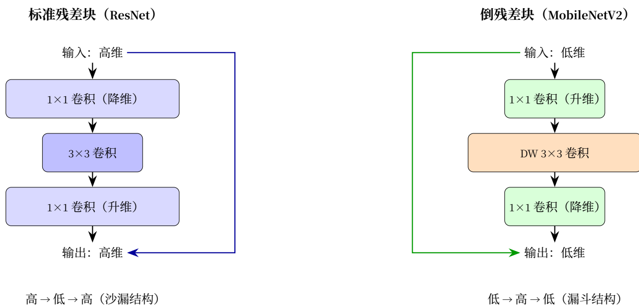
图 34: MobileNetV2 倒残差结构对比
