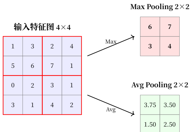
图 6: 2×2 池化操作示意
