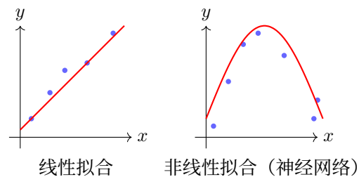
图 5: 从线性到非线性回归
