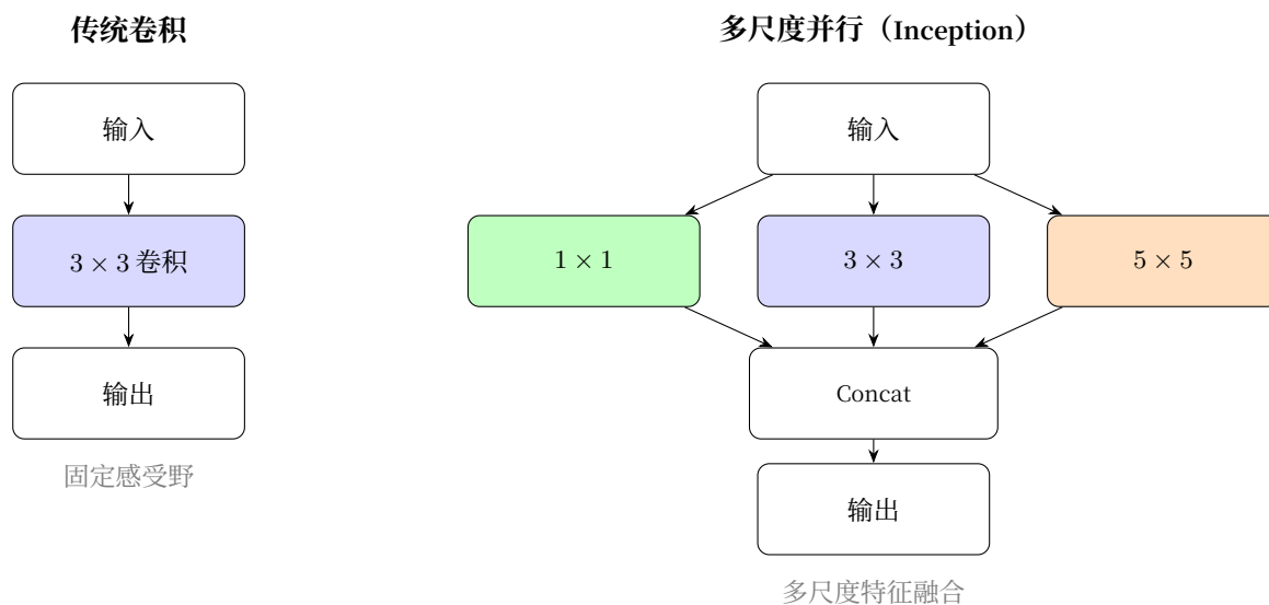
图 29: Inception 的多尺度并行
