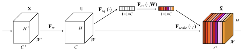
图 20: SE-Net 模块结构: Squeeze → Excite → Scale
