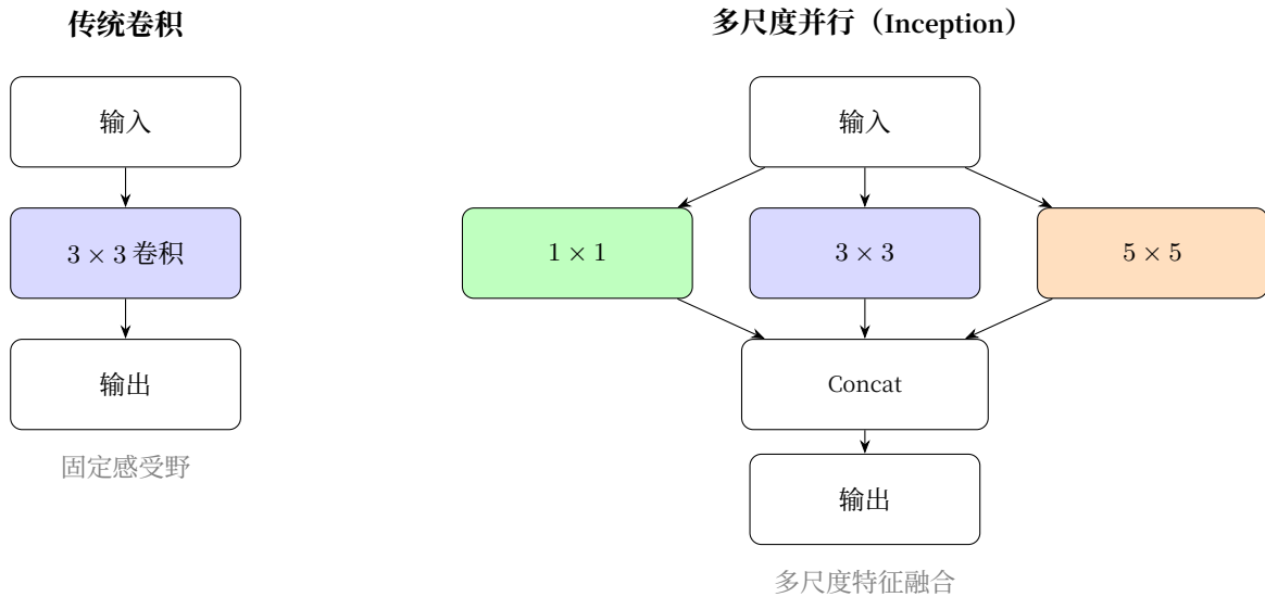
图 2: Inception 的多尺度并行
