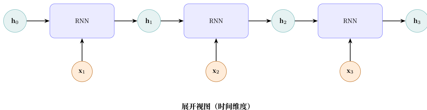
图 1: RNN 循环结构：同一模块在时间上展开
