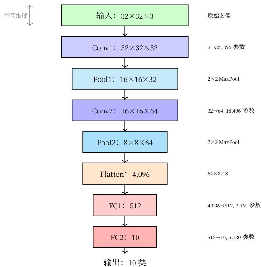
图 1: 基线 CNN 架构: 数据流与参数量
