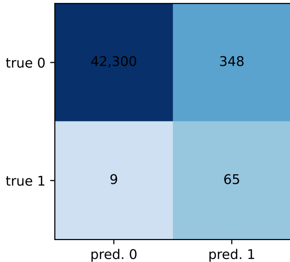
MLP test @0.50 (default)
