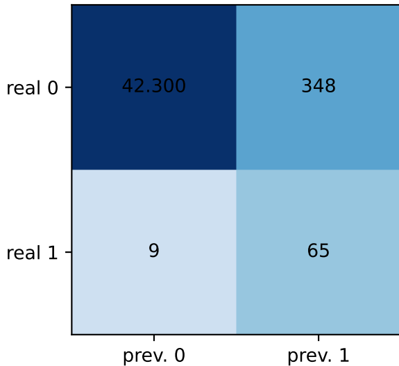
MLP teste @0,50 (default)
