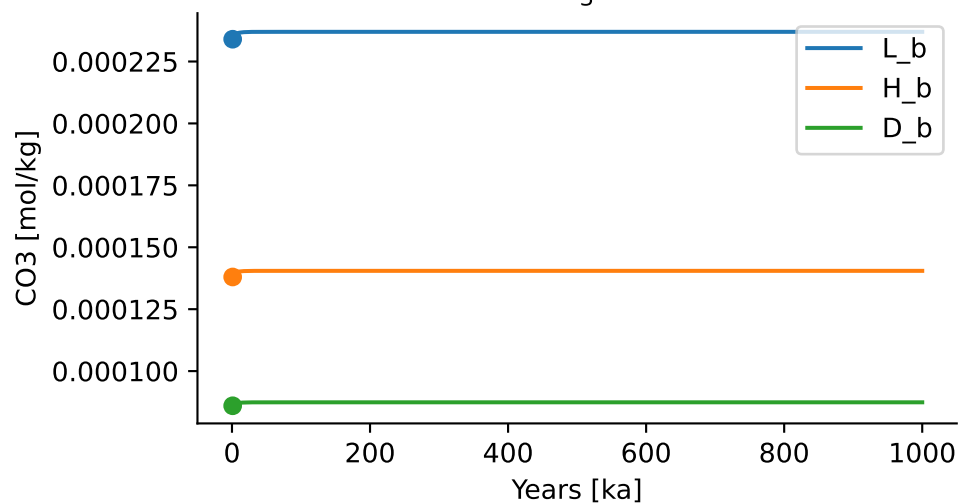
\text{CO}_3^{2-}
