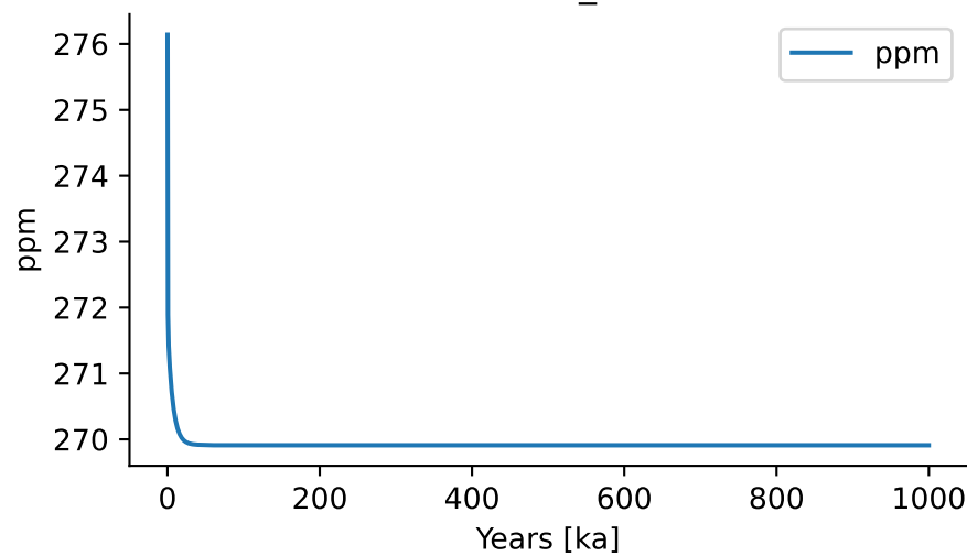
M.CO2_At
