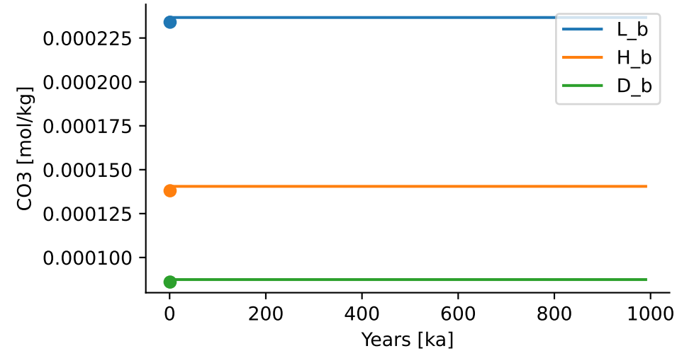
\text{CO}_3^{2-}
