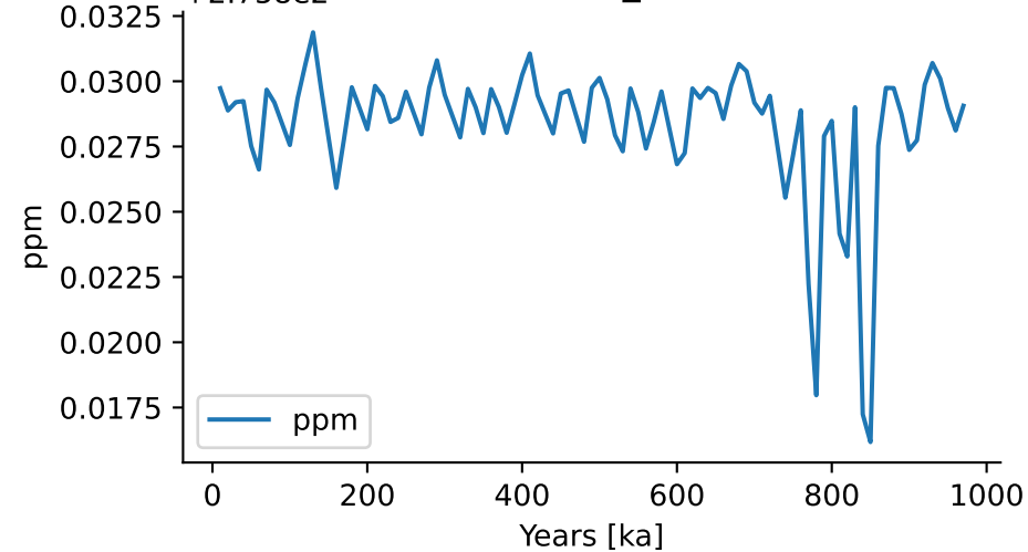
M.CO2_At
