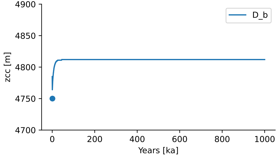
zcc
