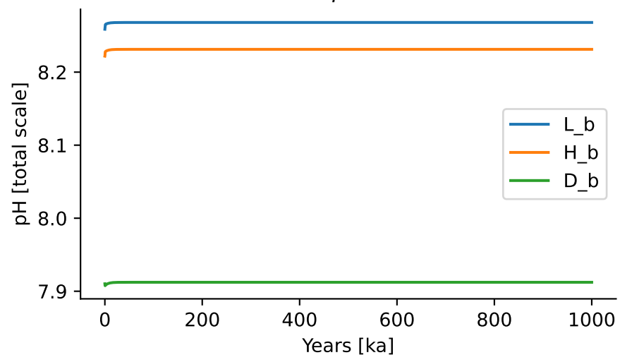
pH
