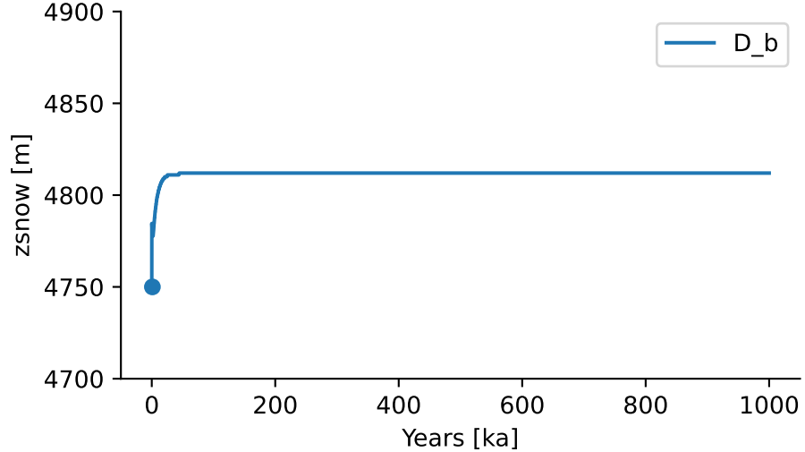
zsnow
