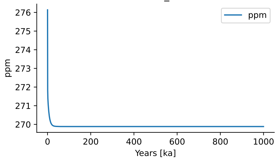
M.CO2_At
