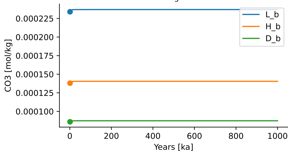
\text{CO}_3^{2-}
