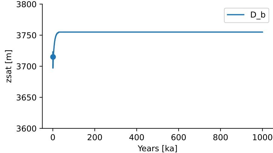
zsat
