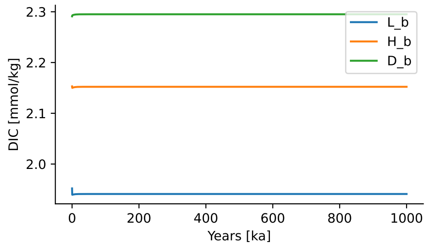
DIC
