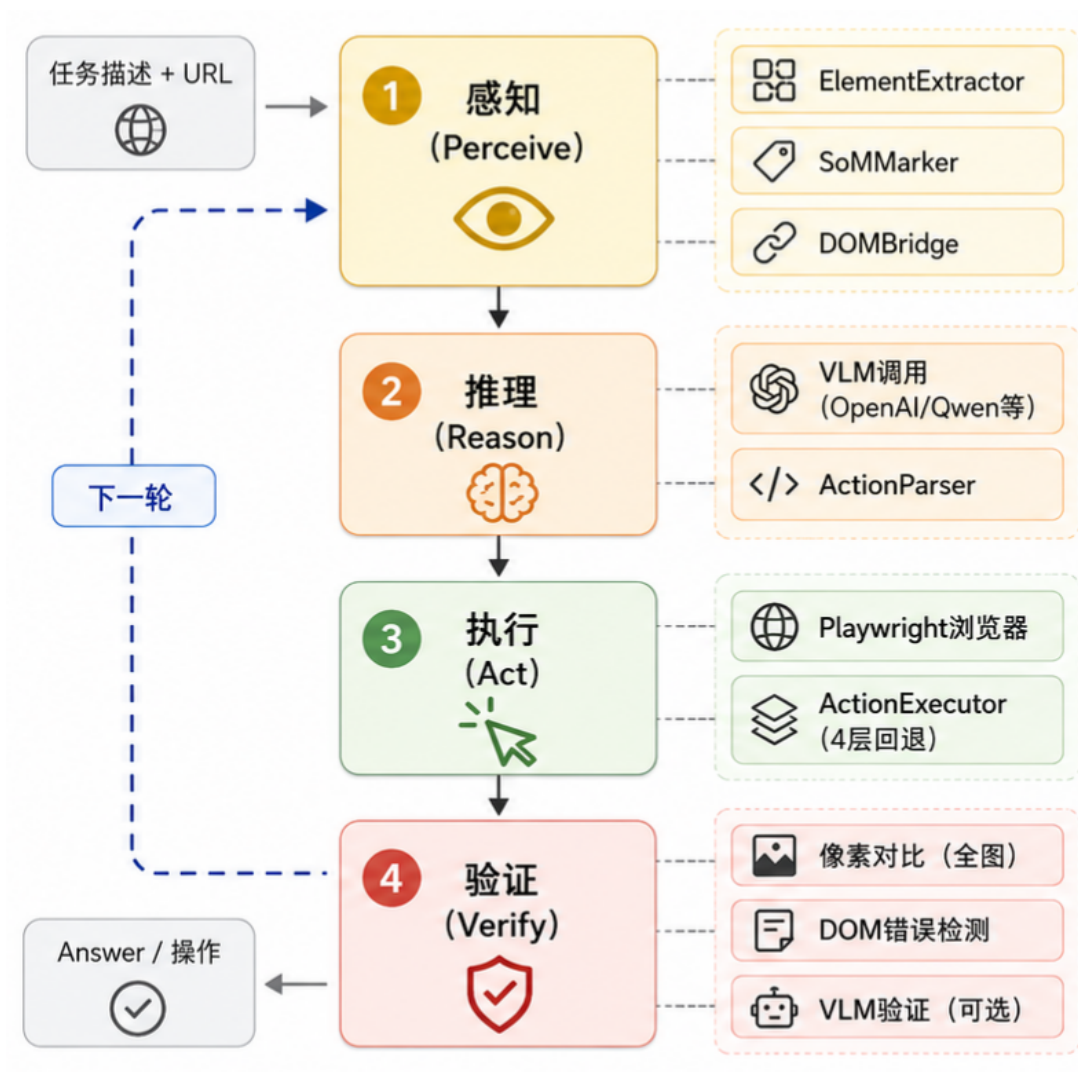
图 1: SoM 视觉输入模式的系统架构
