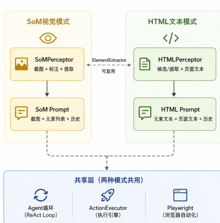
图 3: SoM 模式与 HTML 模式的架构对比
