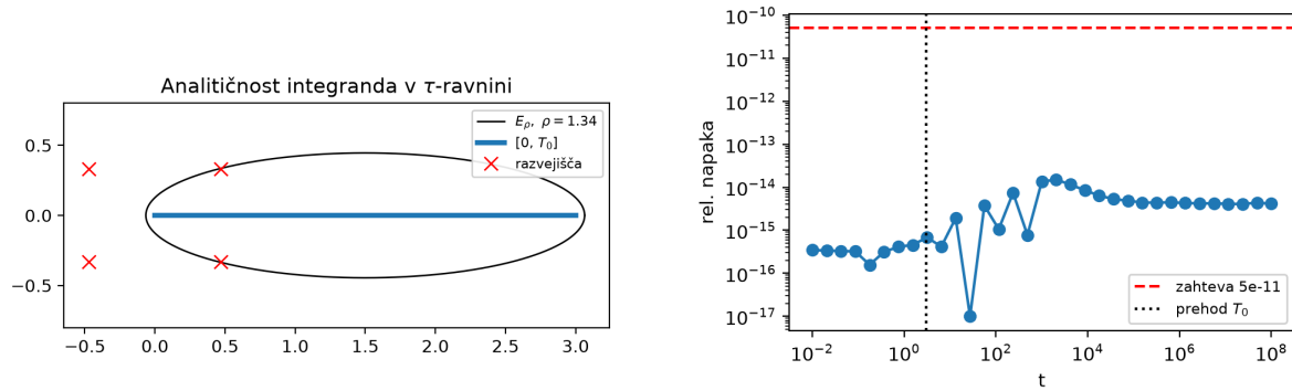
Slika 3: Levo: razvejišča g in Bernsteinova elipsa E_{1,34} za [0, T_0] . Razvejišči, ki sta najbližji elipsi, ležita tik ob robu elipse na desni in določata \rho . Desno: relativna napaka glede na referenco mpmath čez obe veji na 33 točkah med t = 10^{-2} in t = 10^8 . Največja izmerjena napaka je 1,5 \cdot 10^{-14} pri t \approx 2050 , kar je približno 3600-krat pod zahtevanih 5 \cdot 10^{-11} (rdeča črta). Napaka na prehodu pri T_0 (črtna navpičnica) ne izstopa, kar potrjuje, da se veji ujemata gladko. Točka pri t \approx 27 leži na spodnjem robu 10^{-17} , ker je tam odstopanje od reference točno nič.
