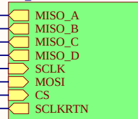
LVDS3 SPI_LVDS.SchDoc
