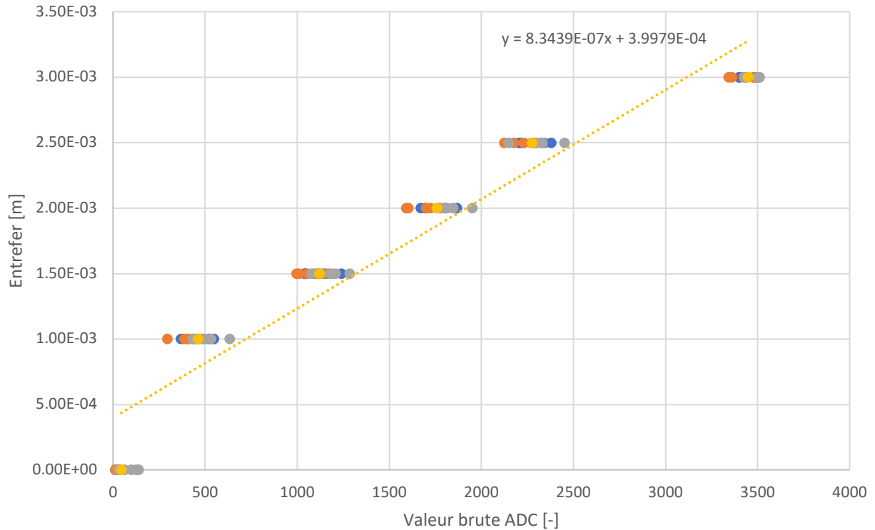
Etalonnage pour l'inducteur 4
