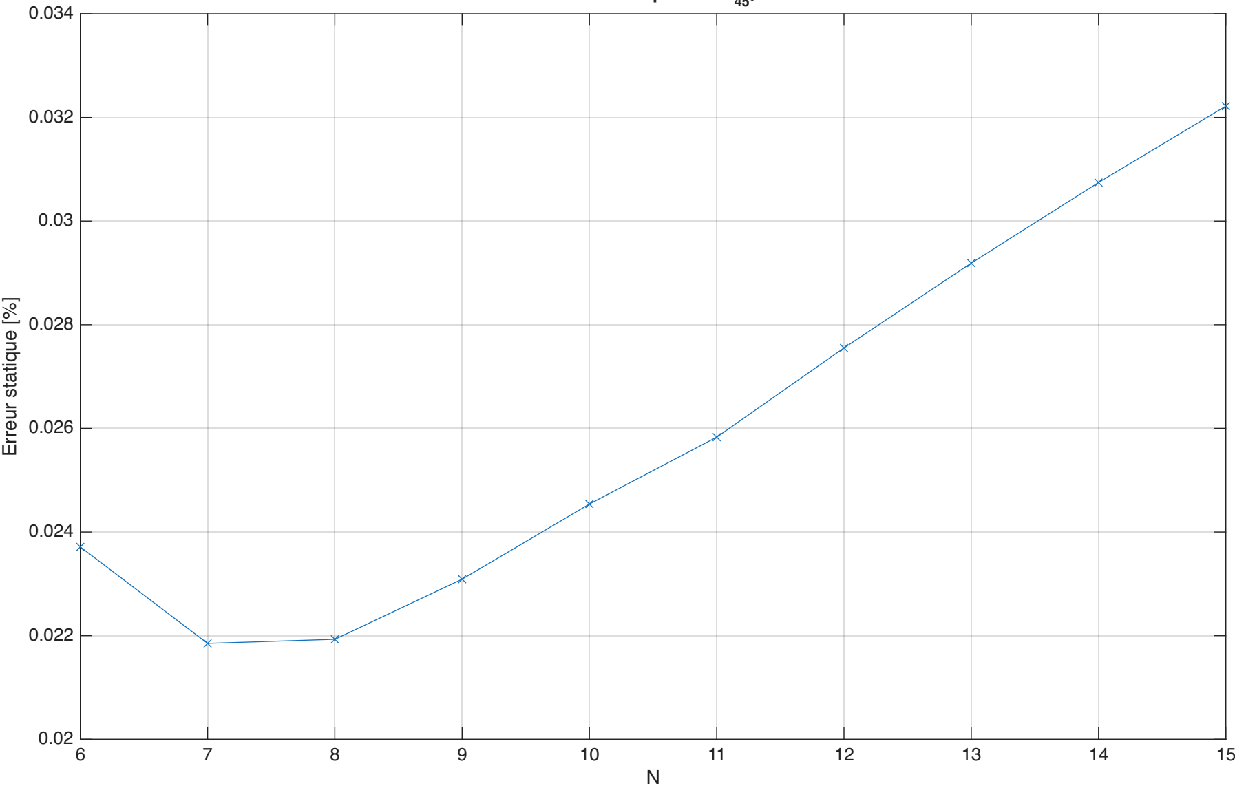
Erreur statique @ m\Phi_{45^\circ}
