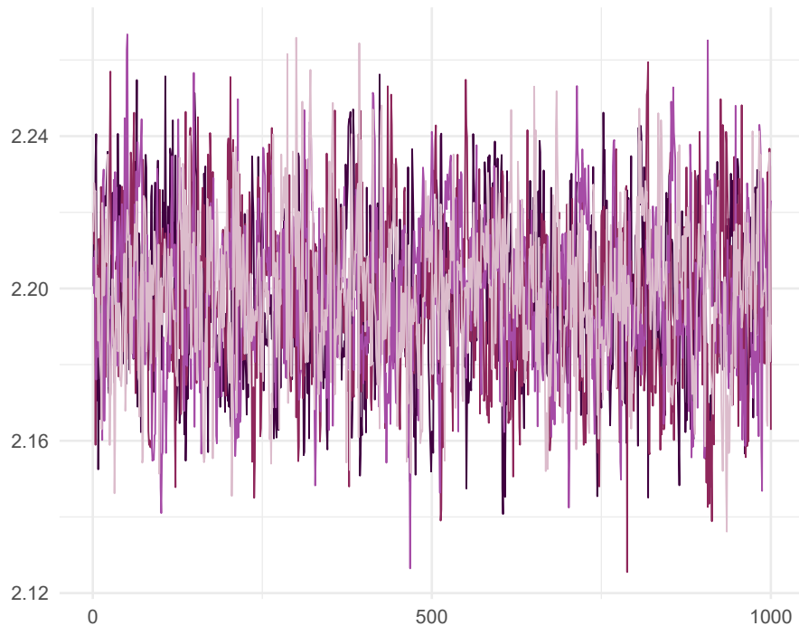
\alpha_0 (Kar-Hamel Mooh)
