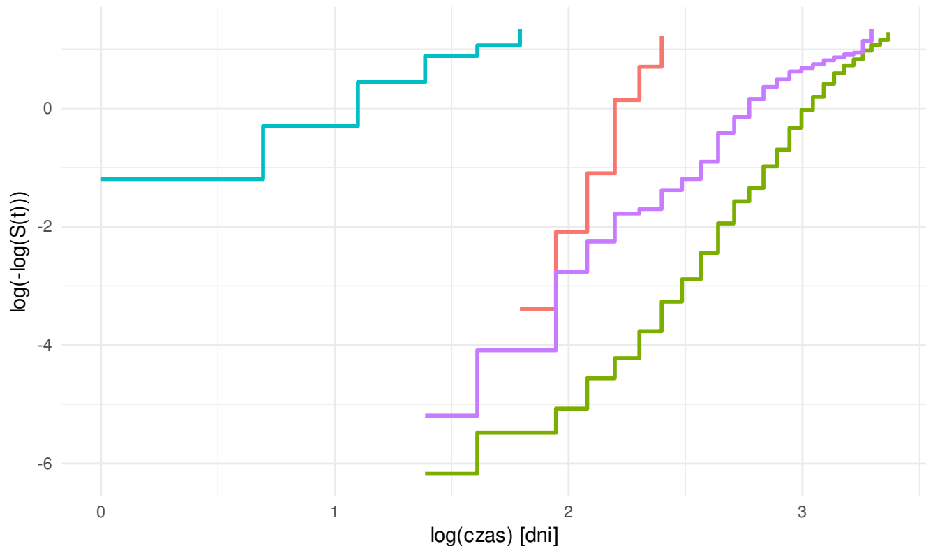
Wykres Complementary Log-Log według grupy związków
