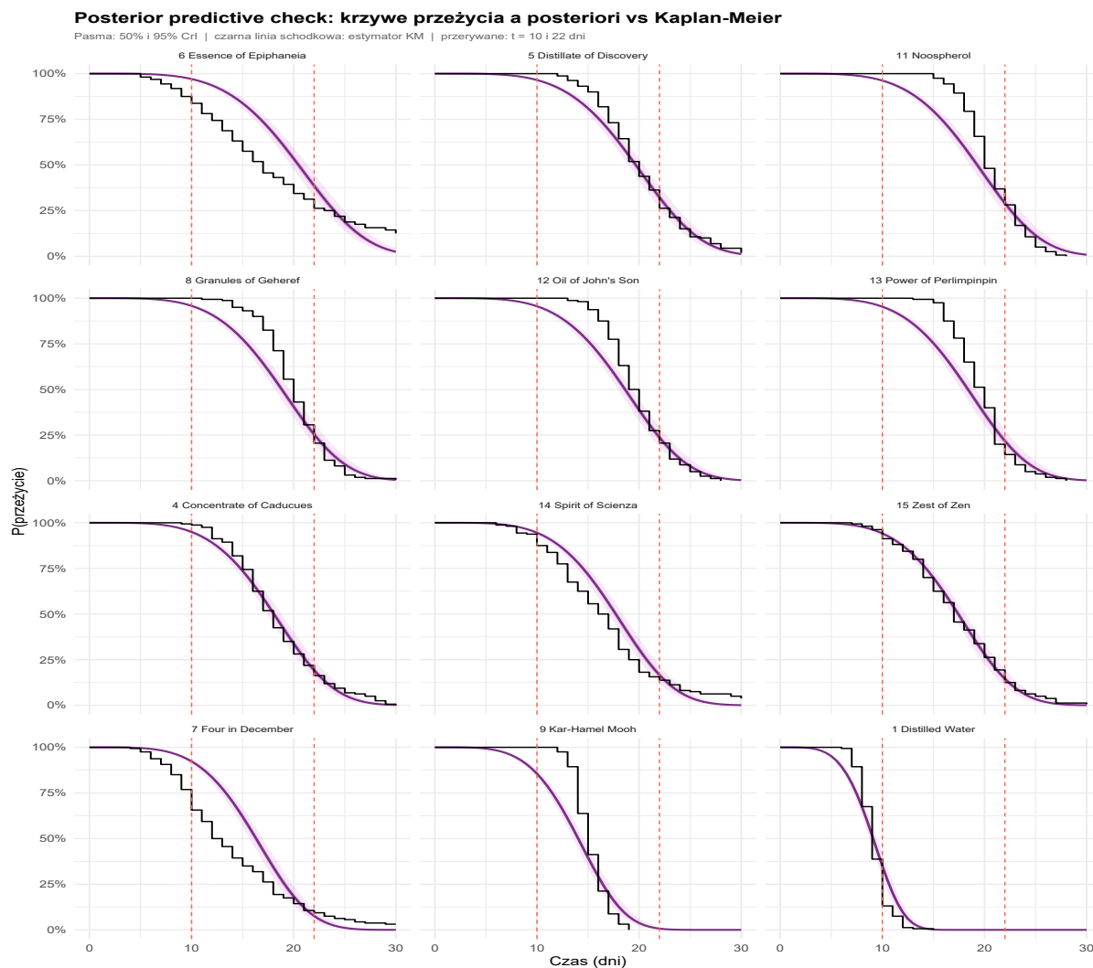
Rycina 4: Posterior predictive check: bayesowskie krzywe przeżycia a posteriori (fioletowe pasma) nałożone na estymator Kaplana-Meiera (czarna linia schodkowa). Uporządkowane według otrzymanego rankingu związków.
