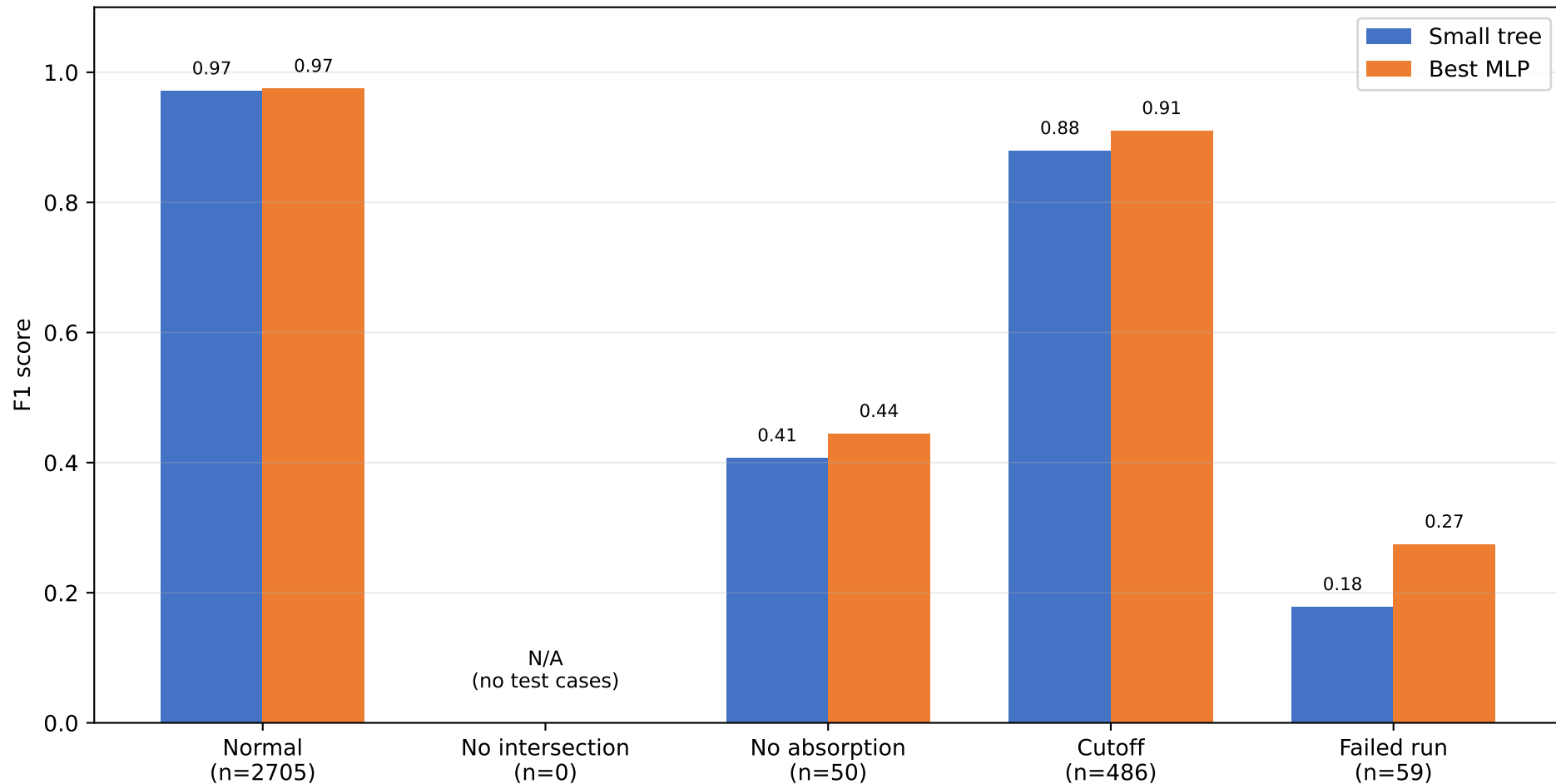
Grouped-label F1 on held-out frames
