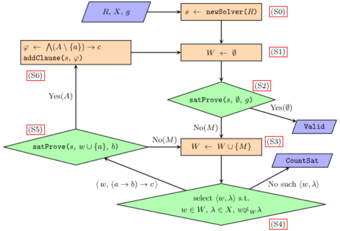
Рисунок 1 — Схема алгоритма proveR с перезапуском
