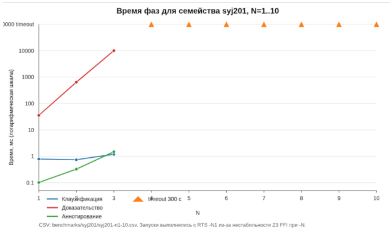
Рисунок 54 — Время фаз разработанного доказателя для N = 1, \dots, 10
