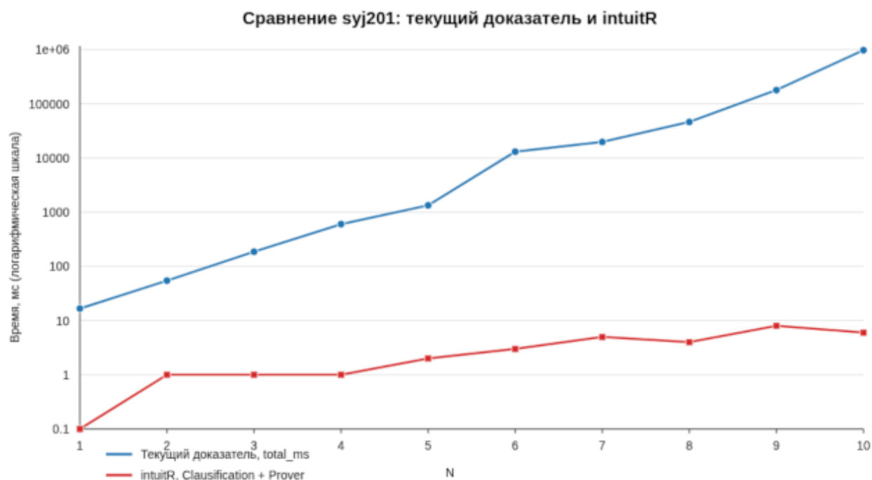
Рисунок 51 — Сравнение полного времени: прототип и intuitR на syj201
