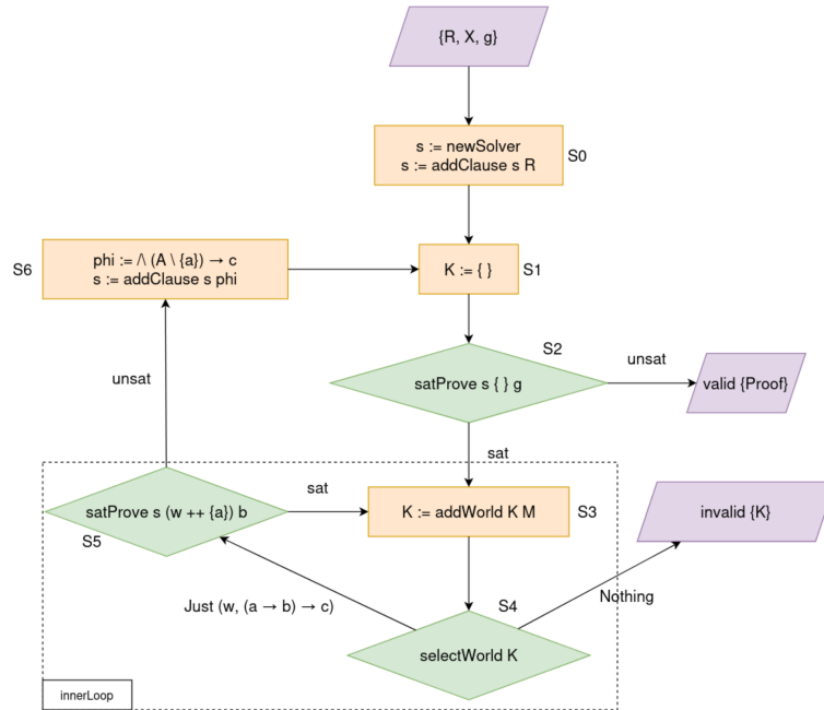
Рисунок 42 — Алгоритм carrow (proveR)
