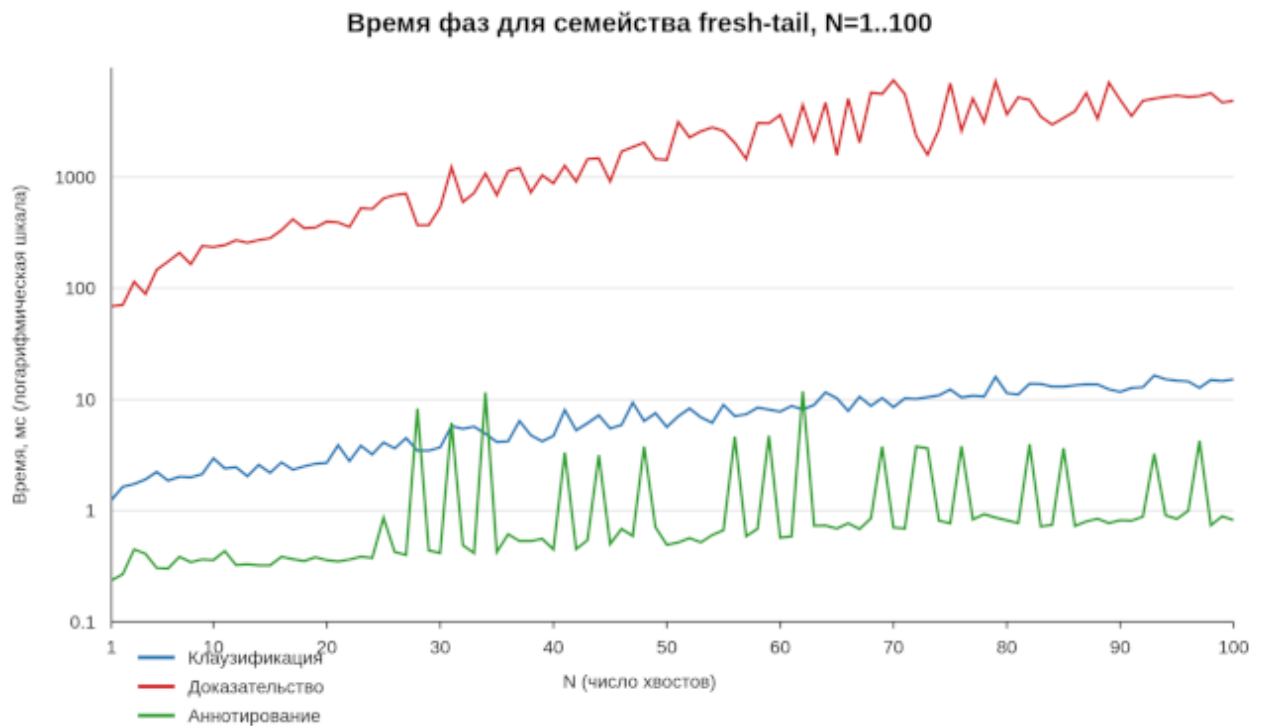
Рисунок 54 — Время фаз прототипа для fresh-tail, N = 1, \dots, 100
