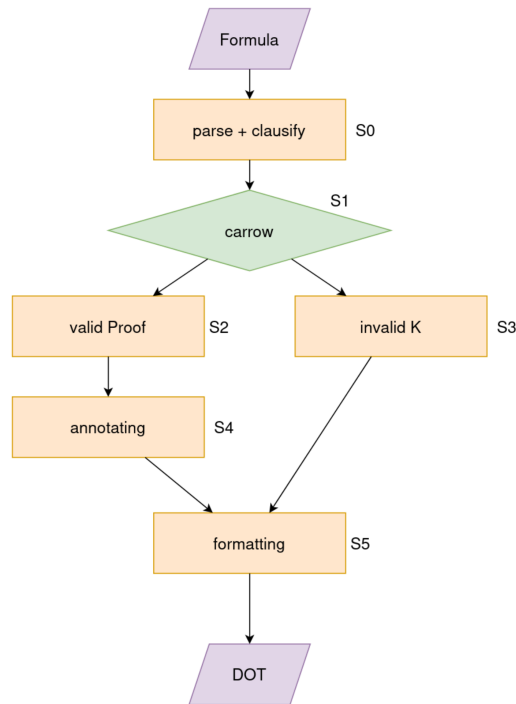
Рисунок 40 — Общая схема конвейера доказательства
