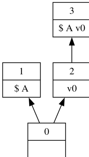
Рисунок 49 — Контрмодель для схемы Пирса
