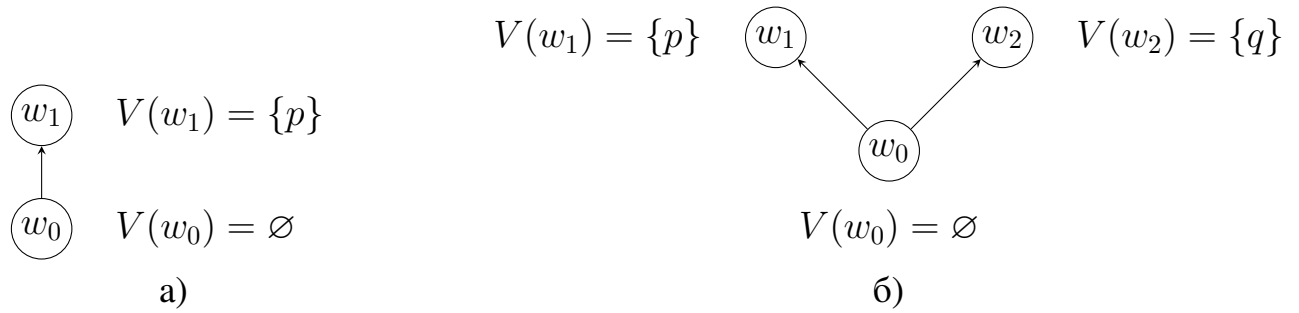
Рисунок 1 — Контрмодели Крипке
