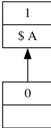
Рисунок 48 — Контрмодель для закона исключённого третьего
