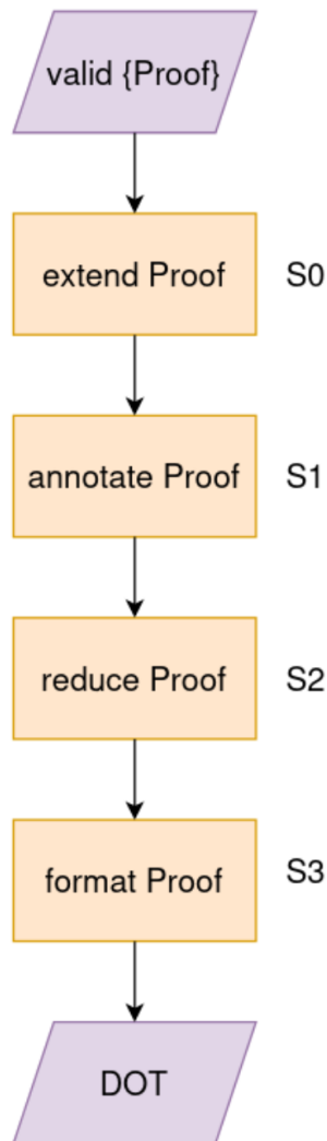
Рисунок 43 — Постобработка успешного доказательства
