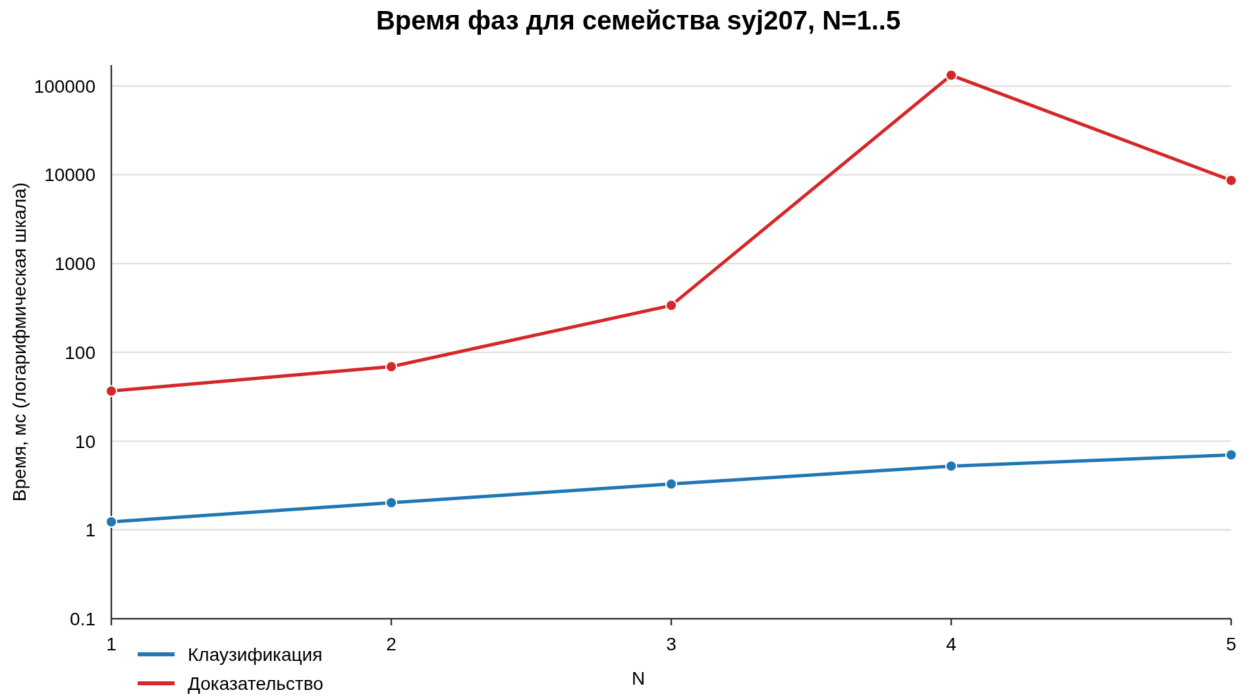
Рисунок 52 — Время фаз прототипа для syj207 , N = 1, \dots, 5
