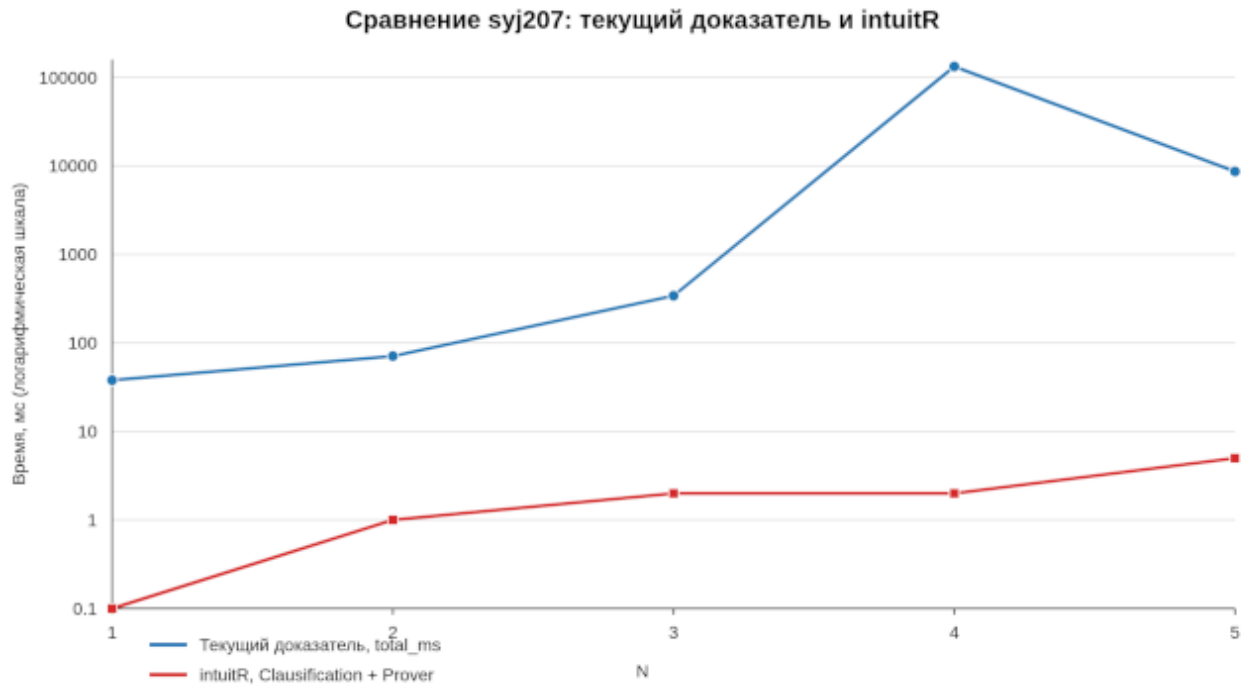
Рисунок 56 — Сравнение полного времени: прототип и intuitR на syj207
