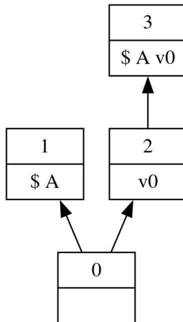
Рисунок 52 — Контрмодель для схемы Пирса
