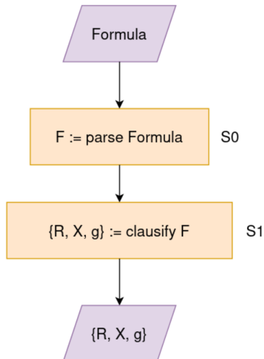
Рисунок 44 — Предобработка формулы перед доказательством
