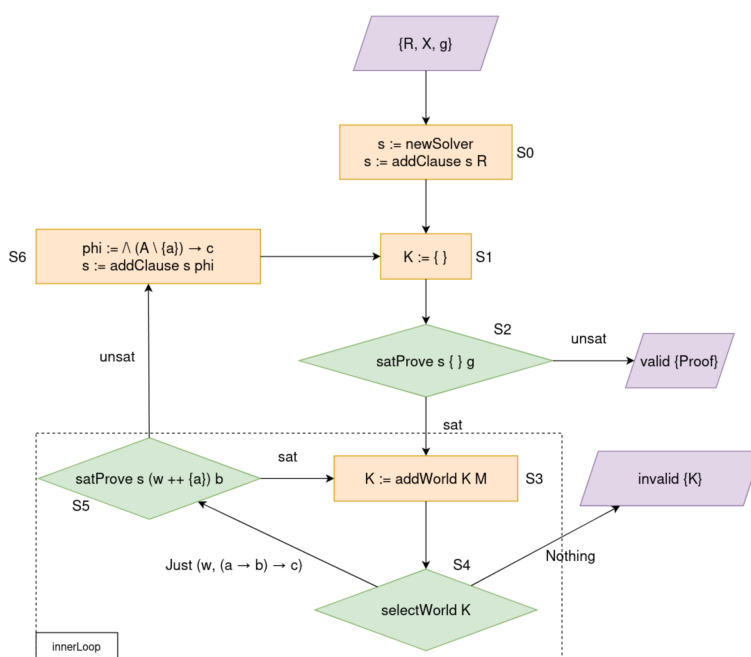
Рисунок 45 — Алгоритм carrow (proveR)
