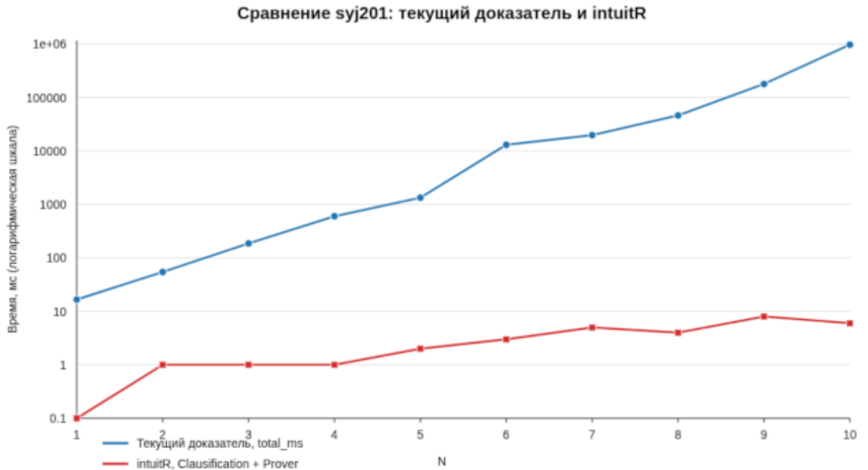
Рисунок 54 — Сравнение полного времени: прототип и intuitR на syj201
