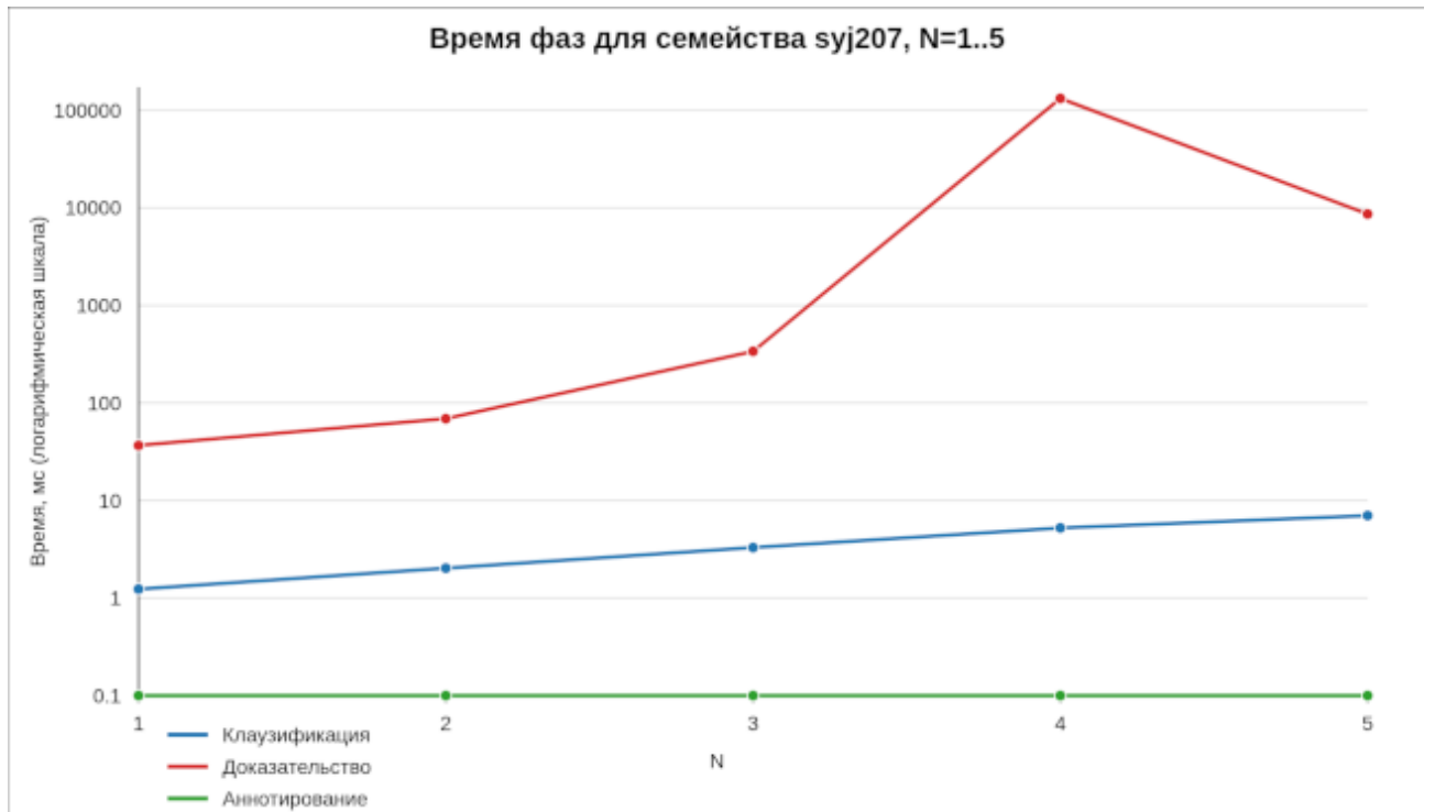
Рисунок 55 — Время фаз прототипа для syj207, N = 1, \dots, 5
