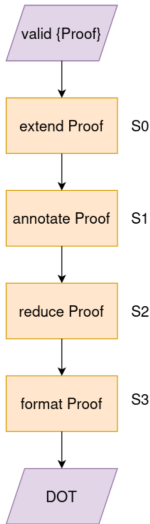
Рисунок 46 — Постобработка успешного доказательства
