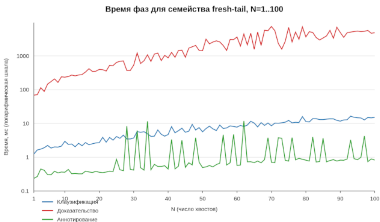
Рисунок 57 — Время фаз прототипа для fresh-tail, N = 1, \dots, 100
