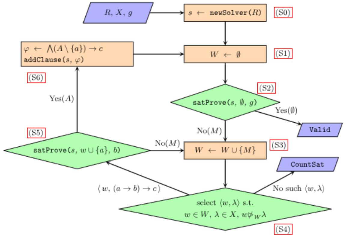
Рисунок 51 — Схема алгоритма proveR с перезапуском
