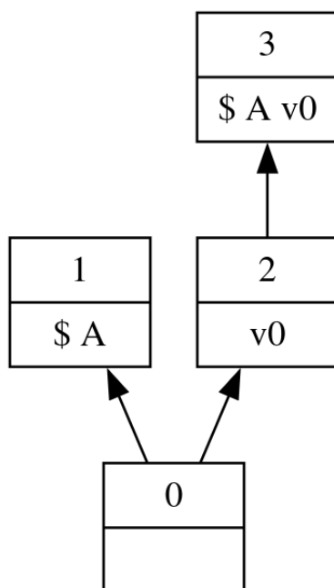
Рисунок 56 — Контрмодель для схемы Пирса
