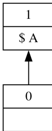
Рисунок 55 — Контрмодель для закона исключённого третьего
