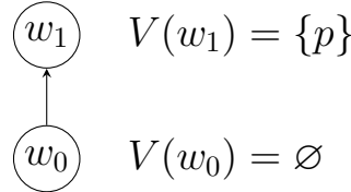
Рисунок 1 — Двухмировая модель Крипке для переменной p
