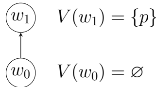
Рисунок 2 — Двухмировая модель Крипке для схемы Пирса
