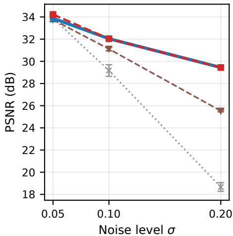
BraTS 2021
