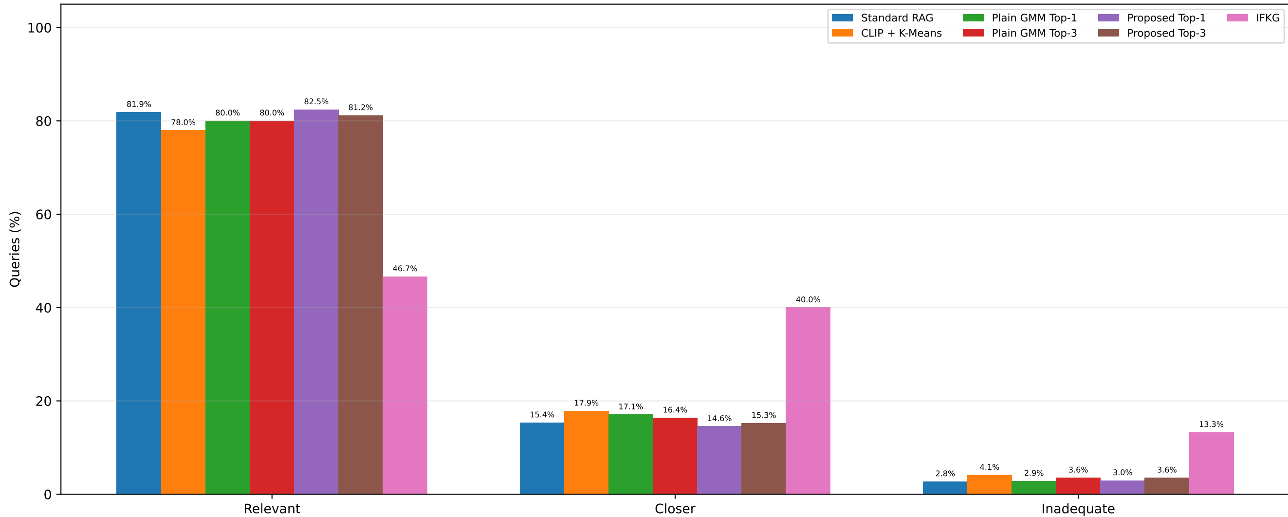
LLM-Judge Evaluation
