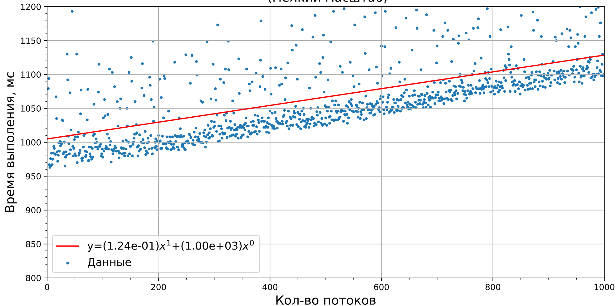
Зависимость времени выполнения алгоритма от количества потоков (мелкий масштаб)
