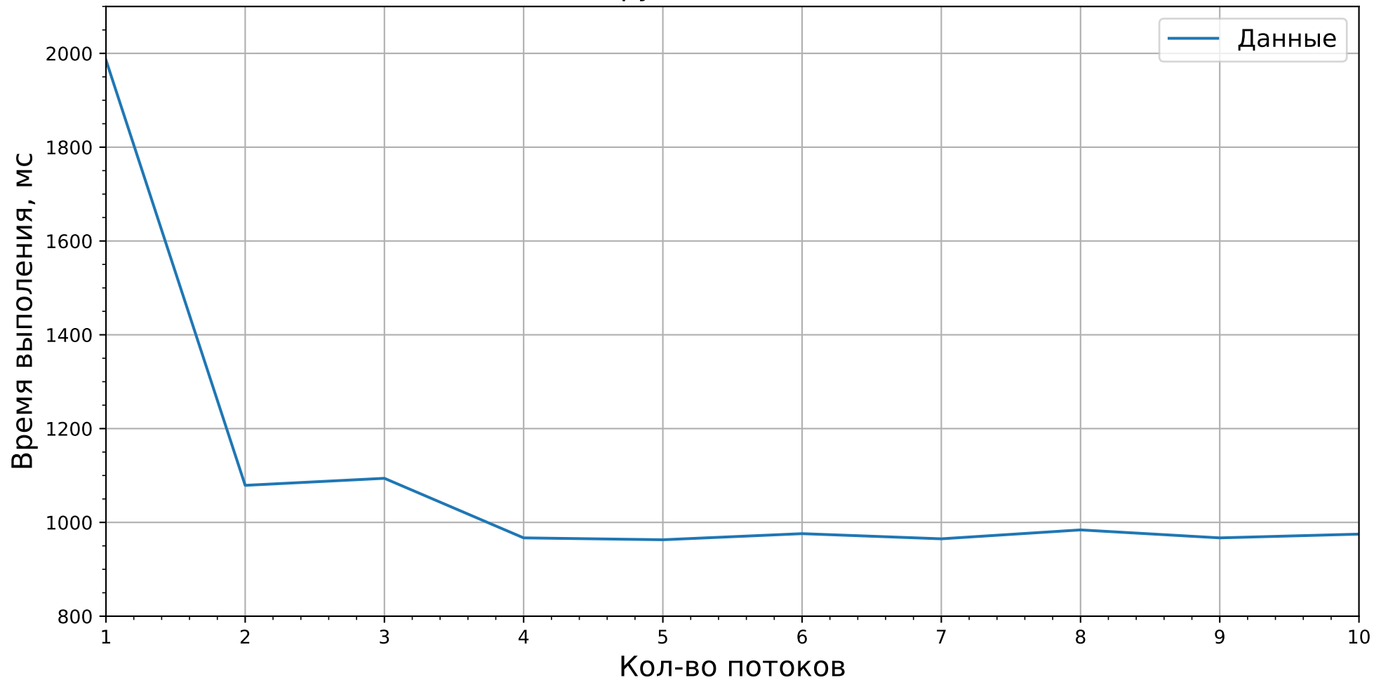
Зависимость времени выполнения алгоритма от количества потоков (крупный масштаб)
