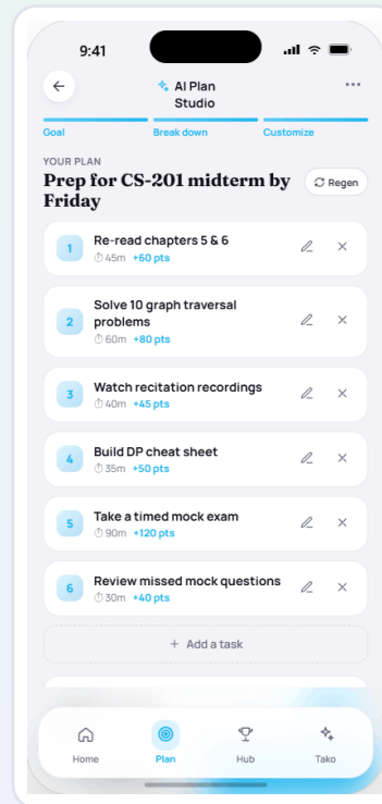
4 · AI Plan
