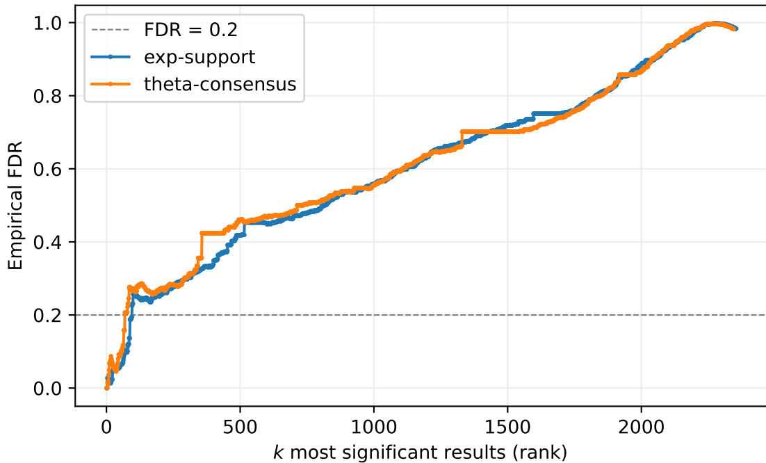
breastCancer sigma=2 theta=0.5
