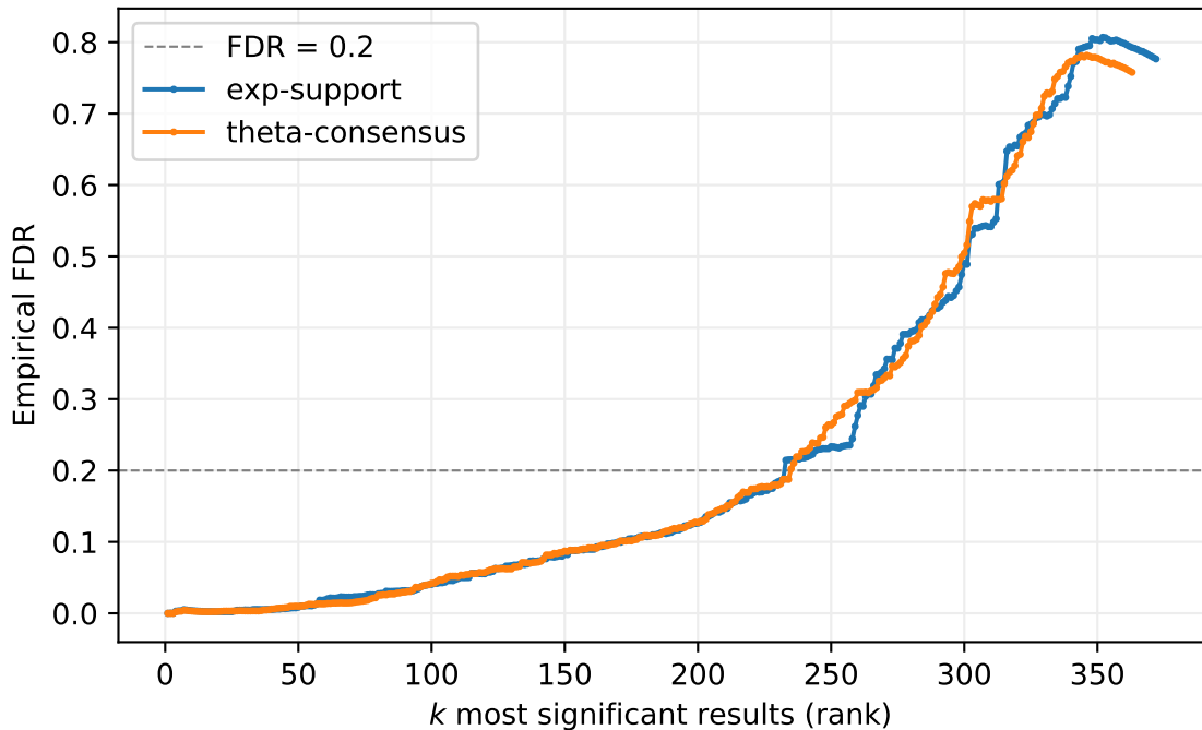
breastCancer sigma=5 theta=1.0
