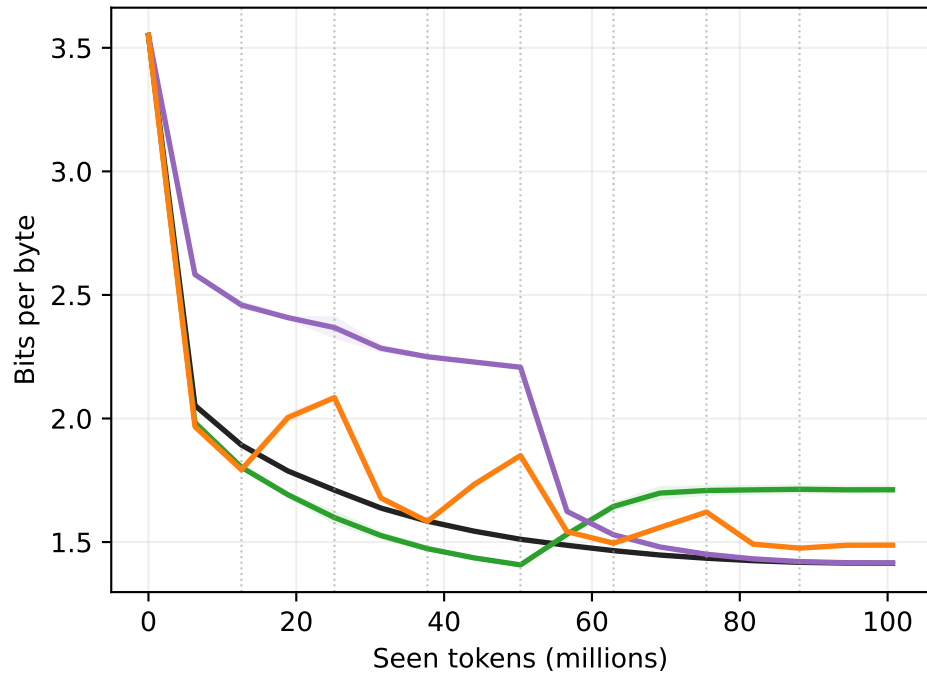
EN order effect
