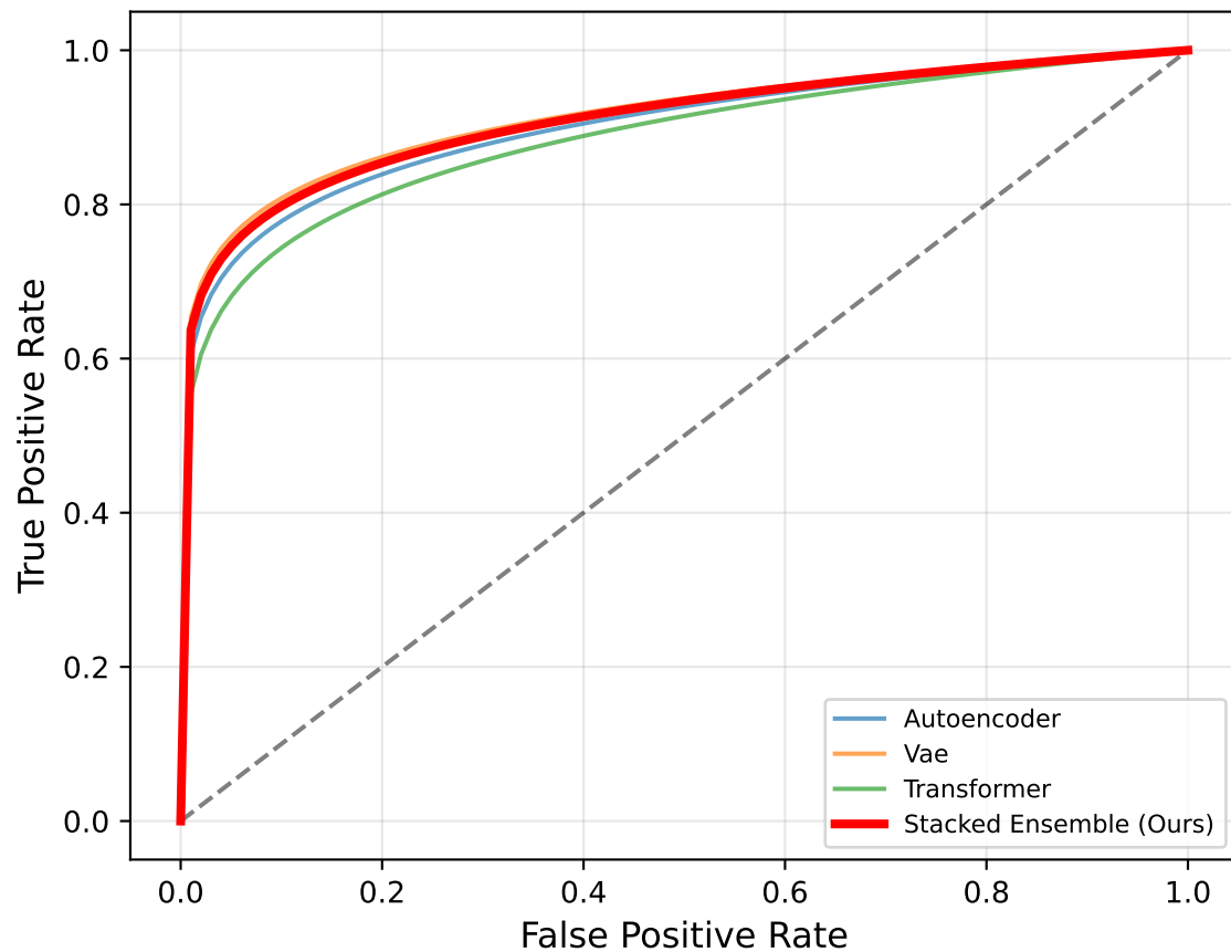
A: Mean ROC Curves
