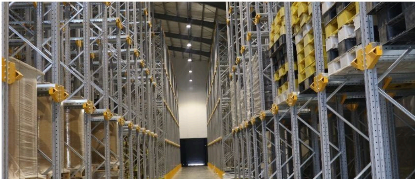
Проезд погрузчика внутри набивного блока, отбойники по низу рам
