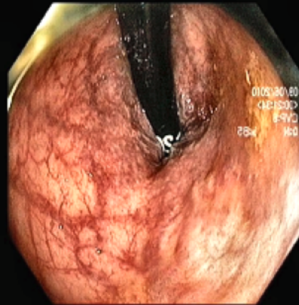
+ Augment
