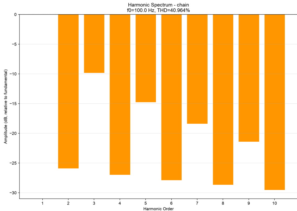
图 15 chain 模型 100 Hz 谐波频谱
