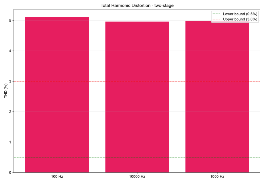
图 14 two-stage 模型 THD 对比
