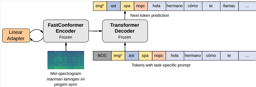
Figura 6: Arquitectura de Canary con Adapters lineales.
