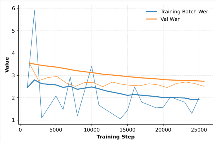
Figura 10: Primera corrida experimental.
