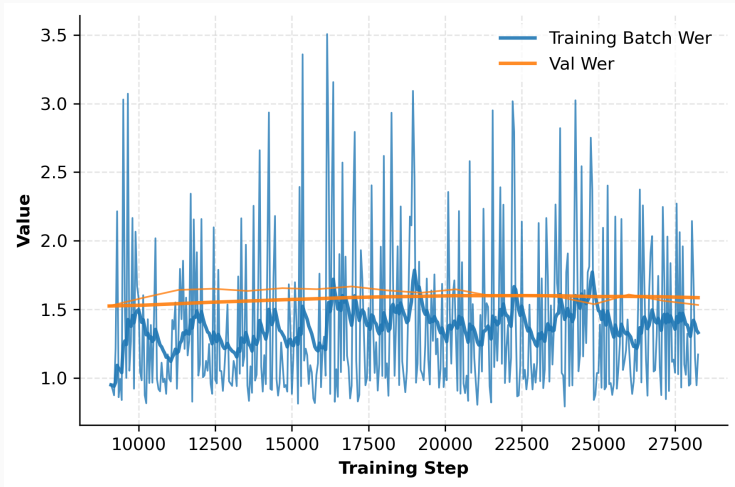
Figura 12: Tercera corrida experimental.
