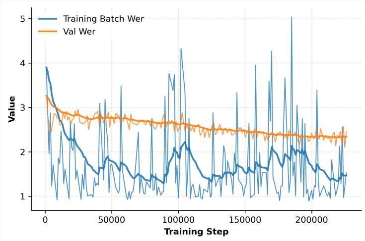
Figura 13: Corrida experimental con audios filtrados y con el modulo de aumentación de datos.
