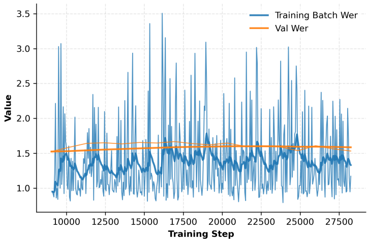
Figura 12: Corrida experimental con audios filtrados.
