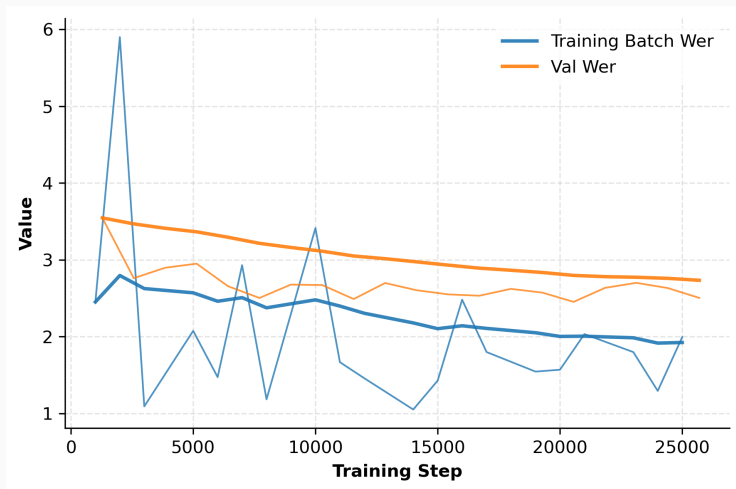
Figura 11: Corrida experimental principal. Incluye el modulo de aumentación de datos.
