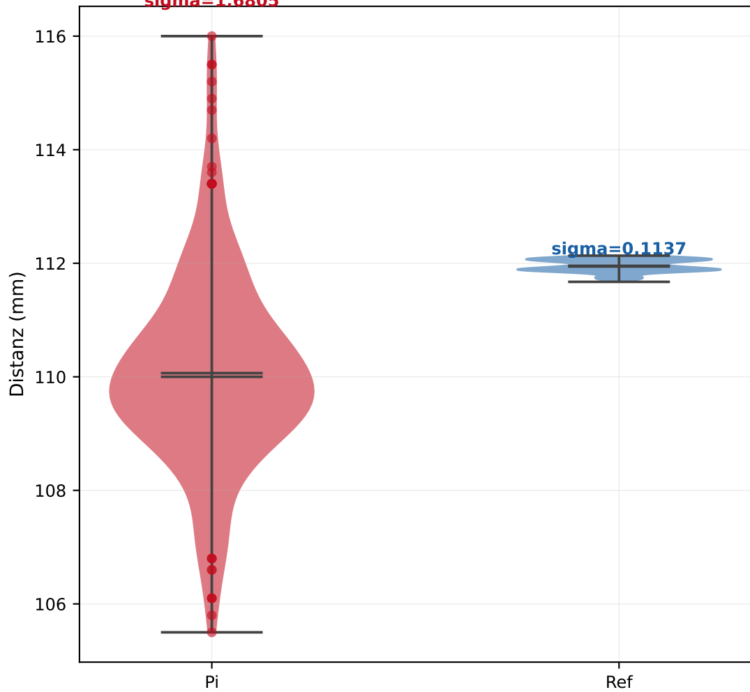
M1 - Verteilung (stationaer)
