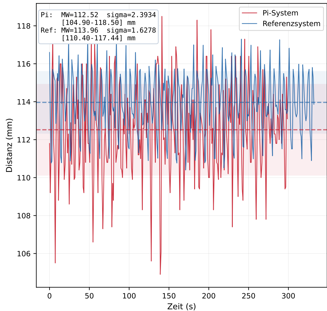
M2 - Zeitverlauf (Zellenrad)
