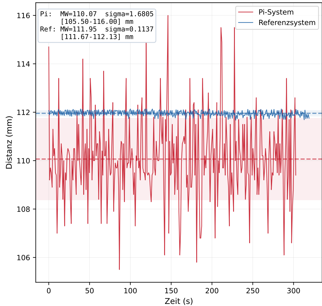
M1 - Zeitverlauf (stationaer)
