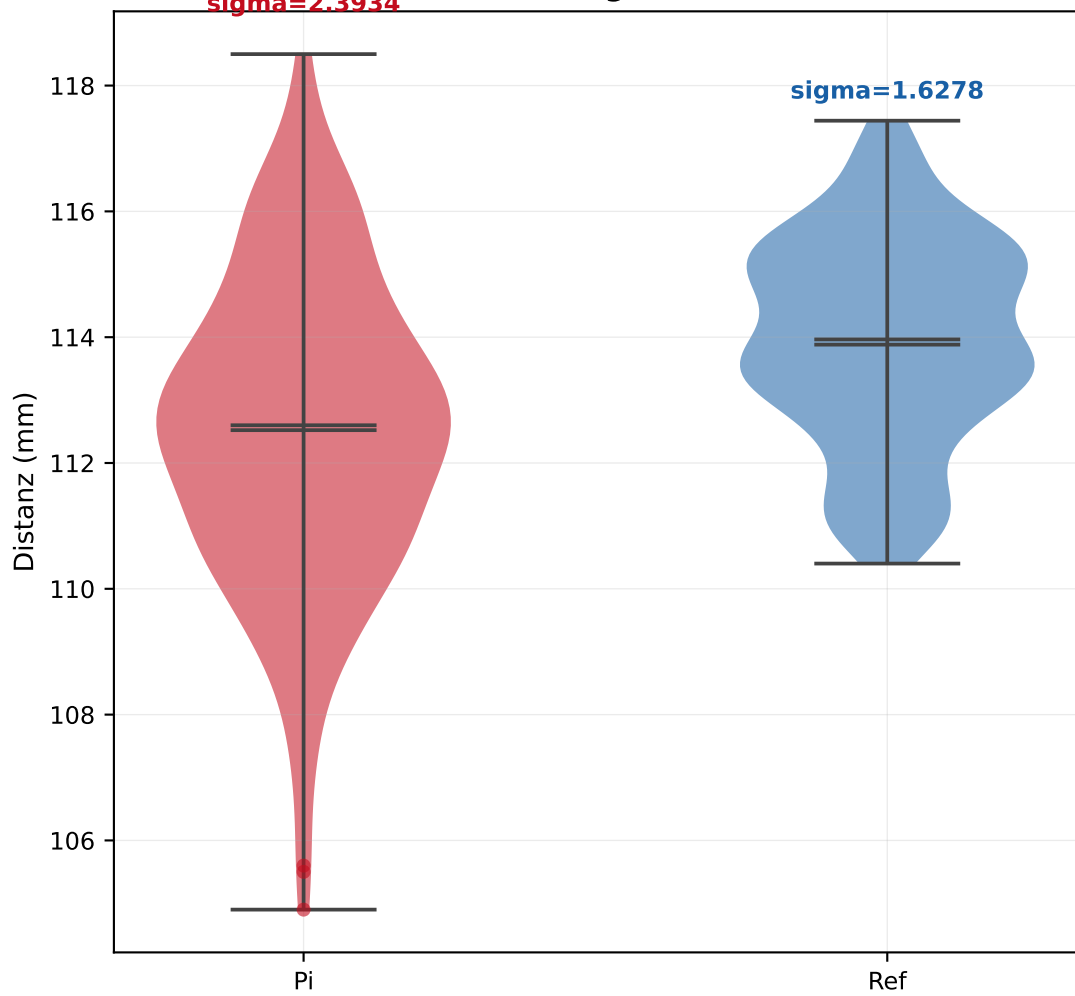
M2 - Verteilung (Zellenrad)
