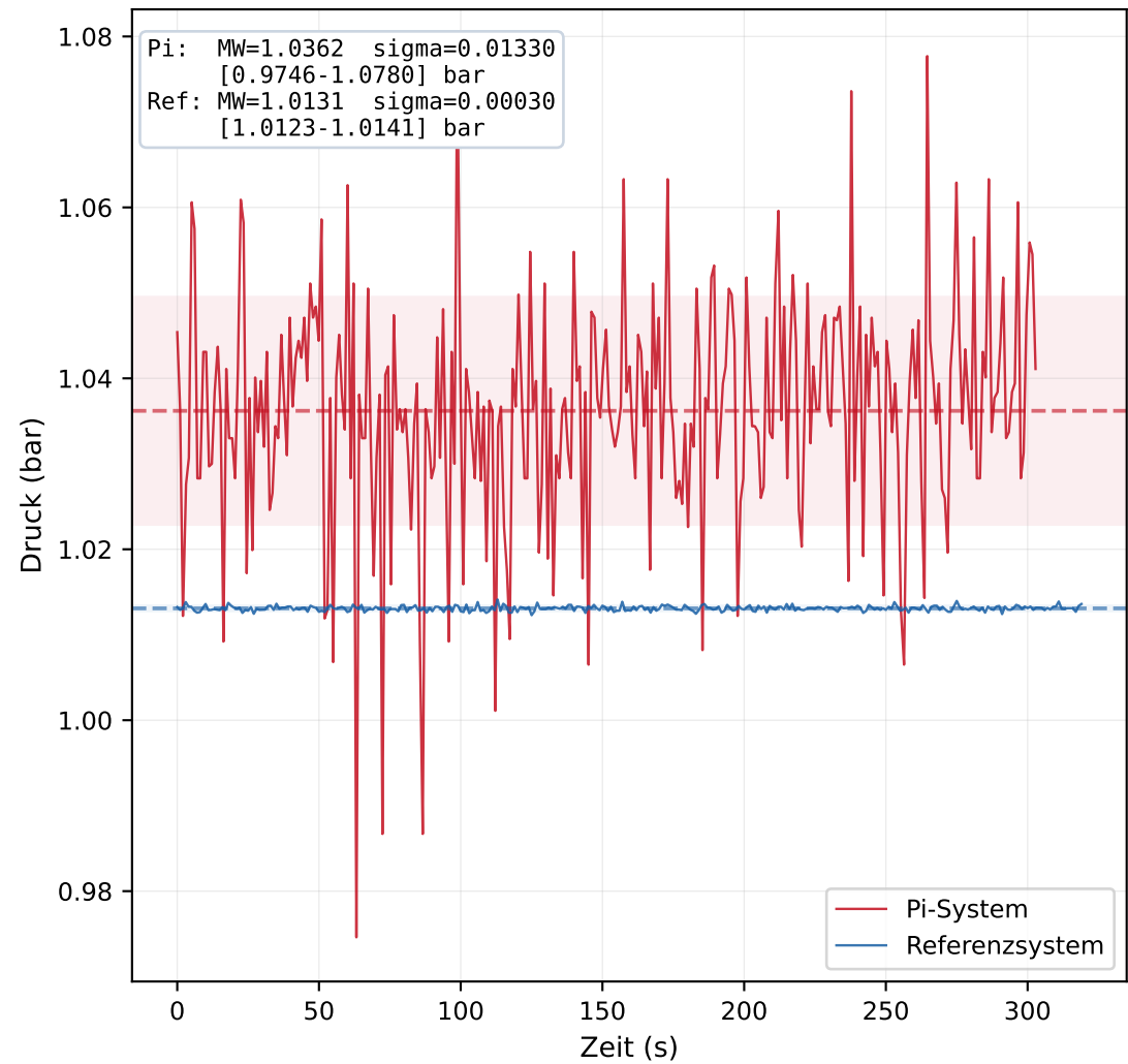
M1 - Zeitverlauf (Atmosphaerendruck)
