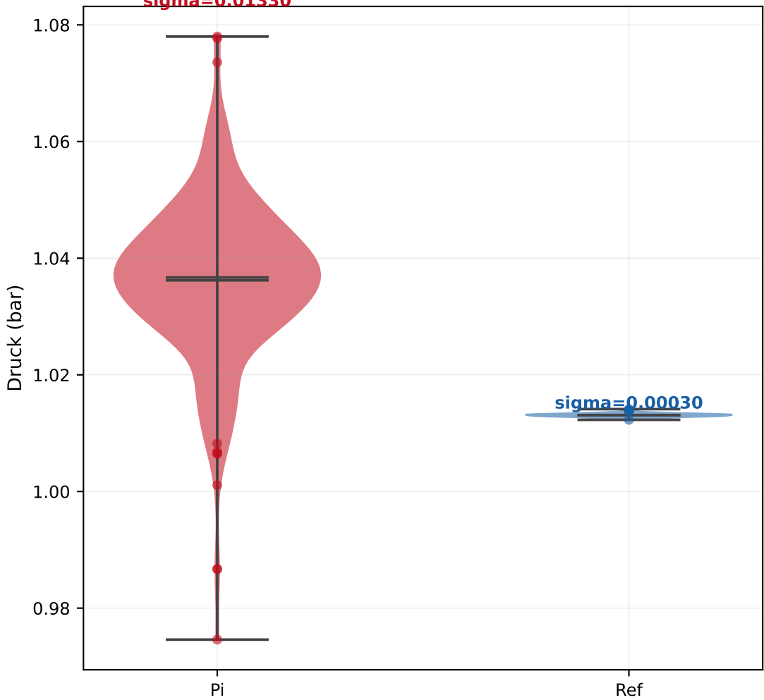
M1 - Verteilung (Atmosphaerendruck)
