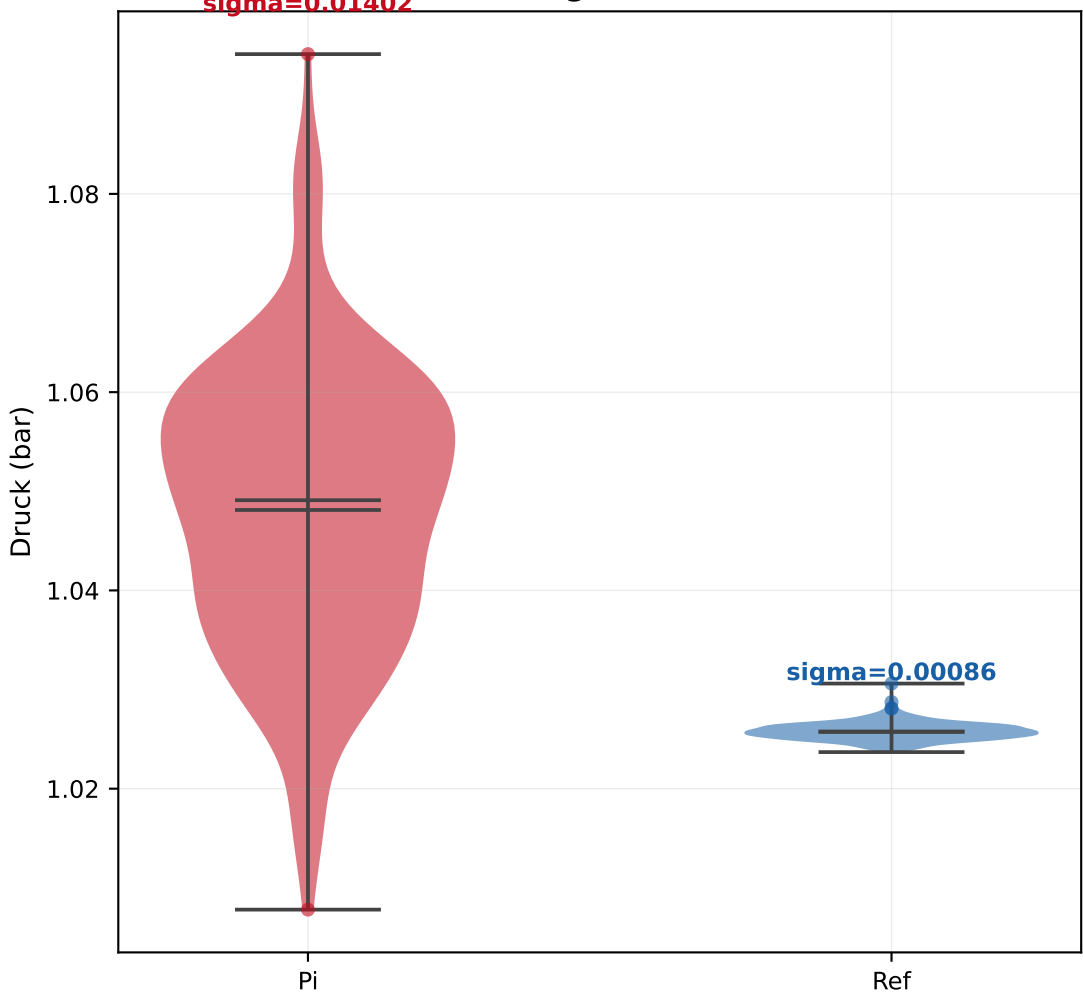
M2 - Verteilung (Geblaease aktiv)
