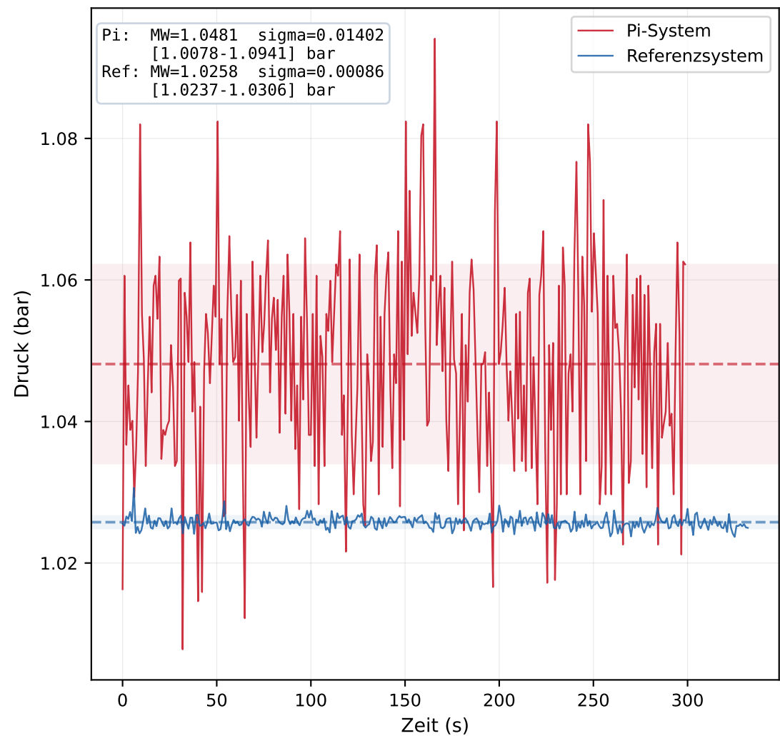
M2 - Zeitverlauf (Geblaease aktiv)
