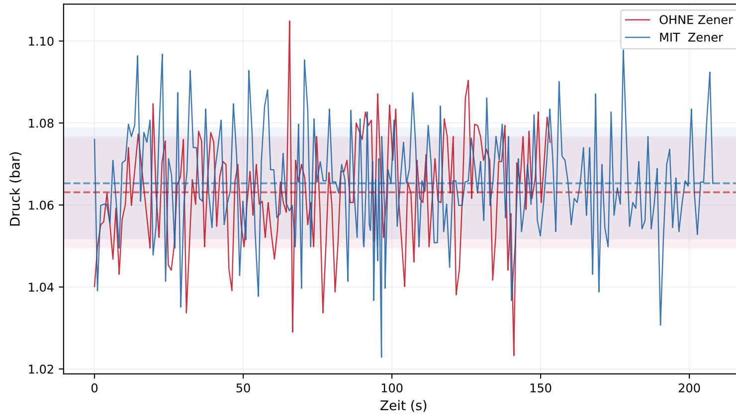
Drucksensor - Zeitverlauf
