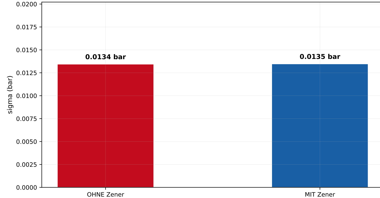
Drucksensor - Standardabweichung
