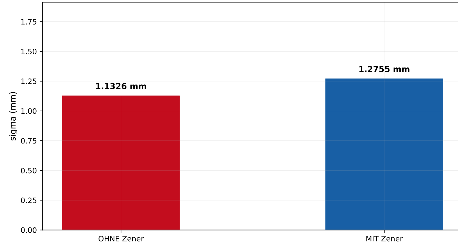
Distanzsensor - Standardabweichung
