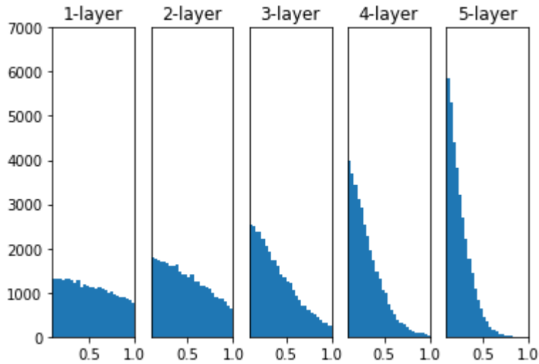
LeCun
