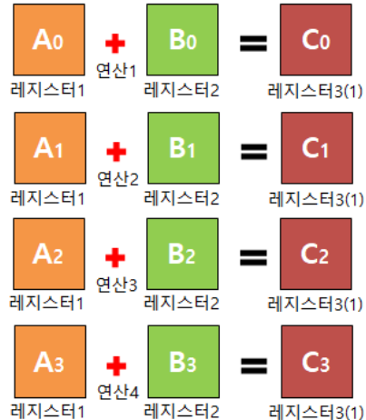
SISD 연산
