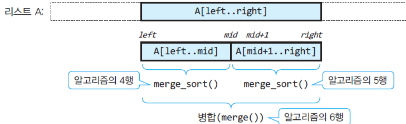
[그림 5.4] 알고리즘 5.1의 구조
