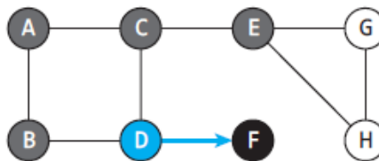
(e) D → F 큐 내용: EF
