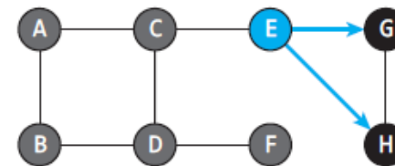
(f) E → G, H 큐 내용: FGH
