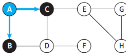
(b) A → B, C 큐 내용: BC
