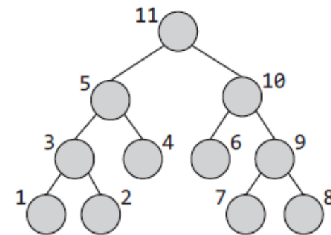
후위 순회: LRV
