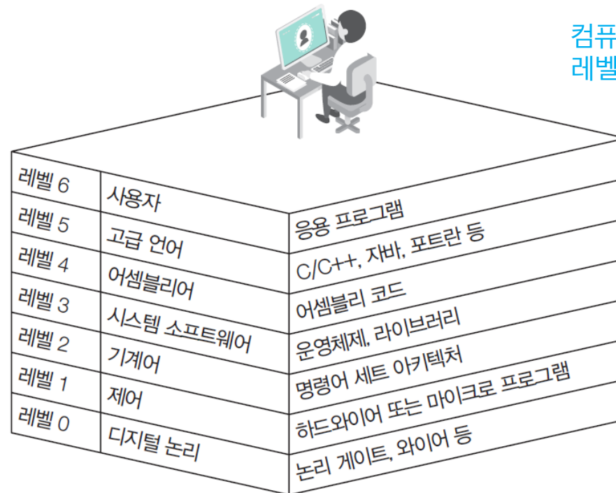
그림 1-8 컴퓨터 시스템의 추상화 레벨
