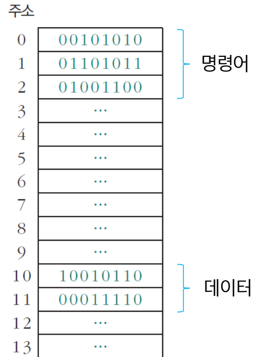
그림 1-7 프로그램과 데이터가 주기억 장치에 저장되어 있는 예
