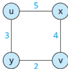
가중치 그래프
