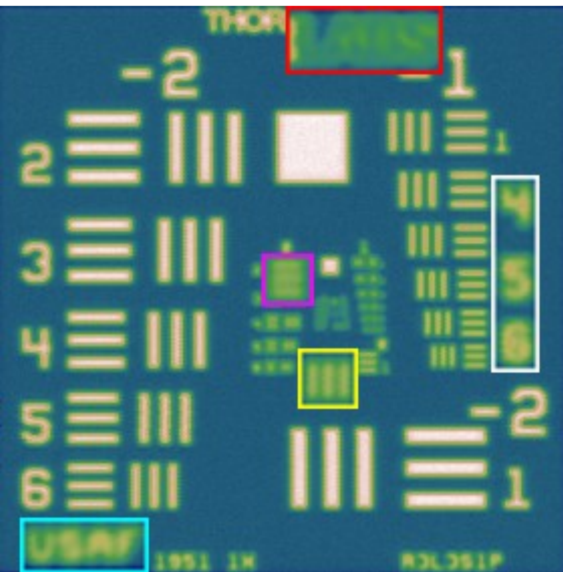
(a) I_{1.5}
