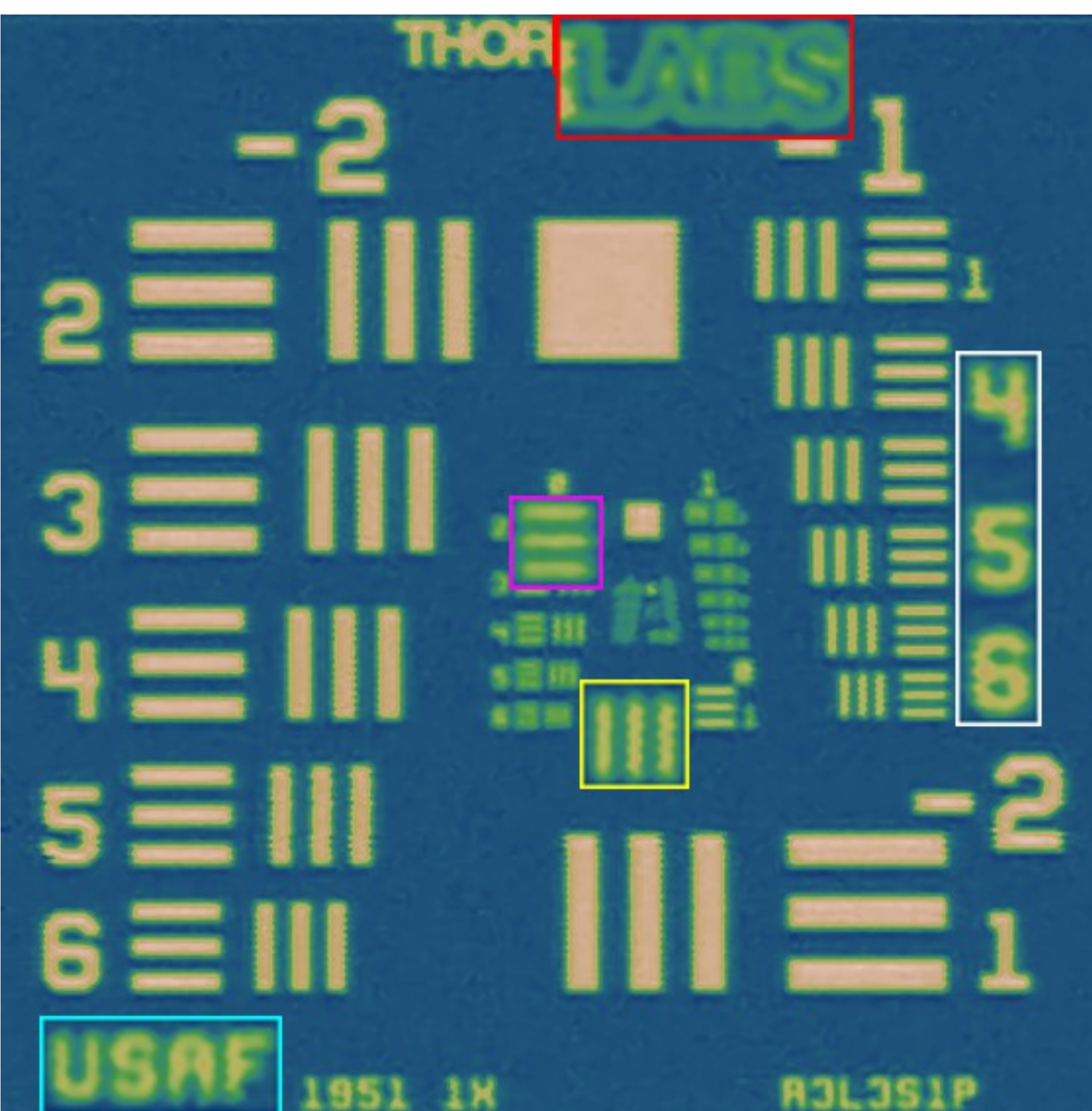
(d) NAFNetSR
