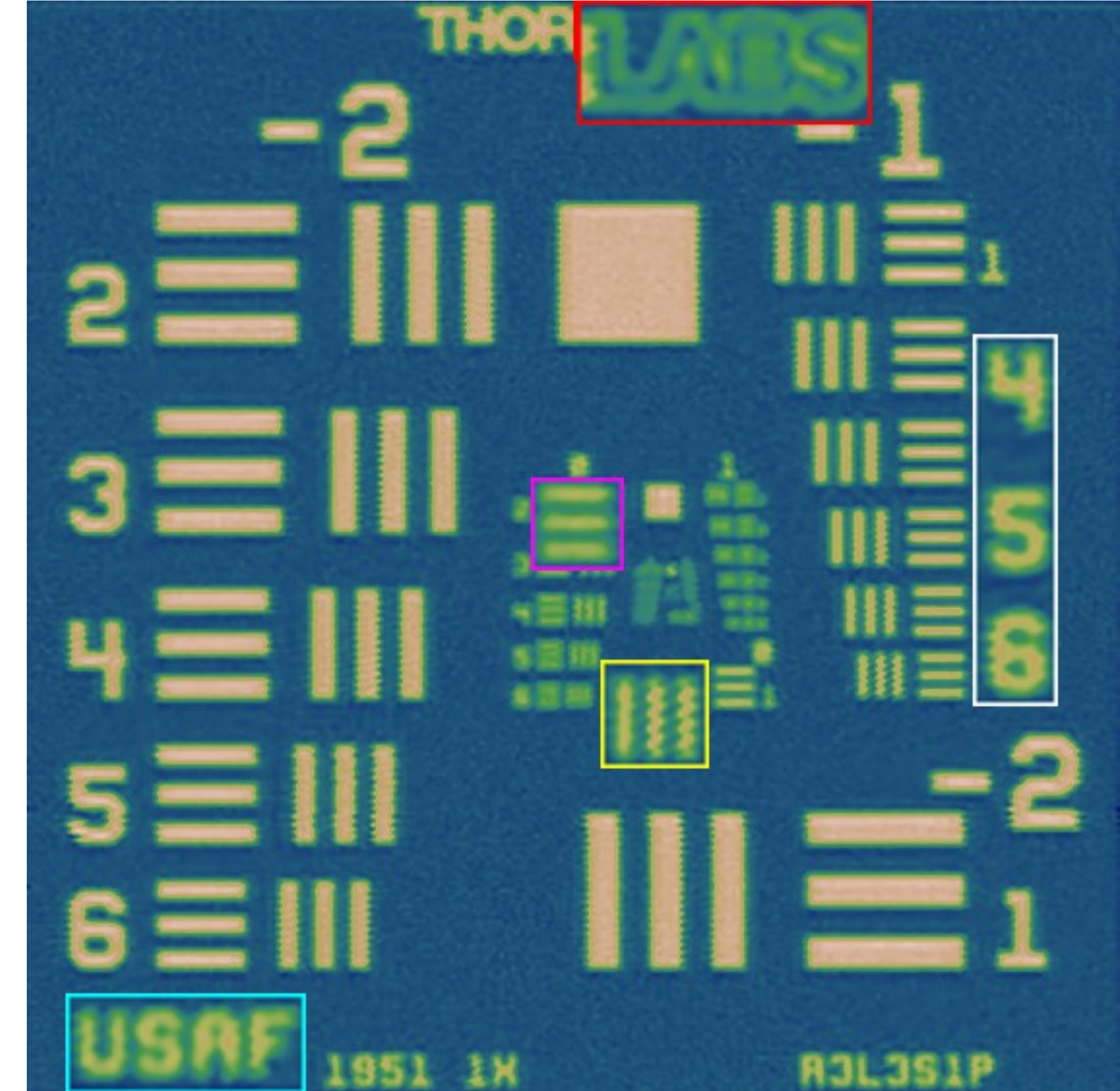
(c) HAN
