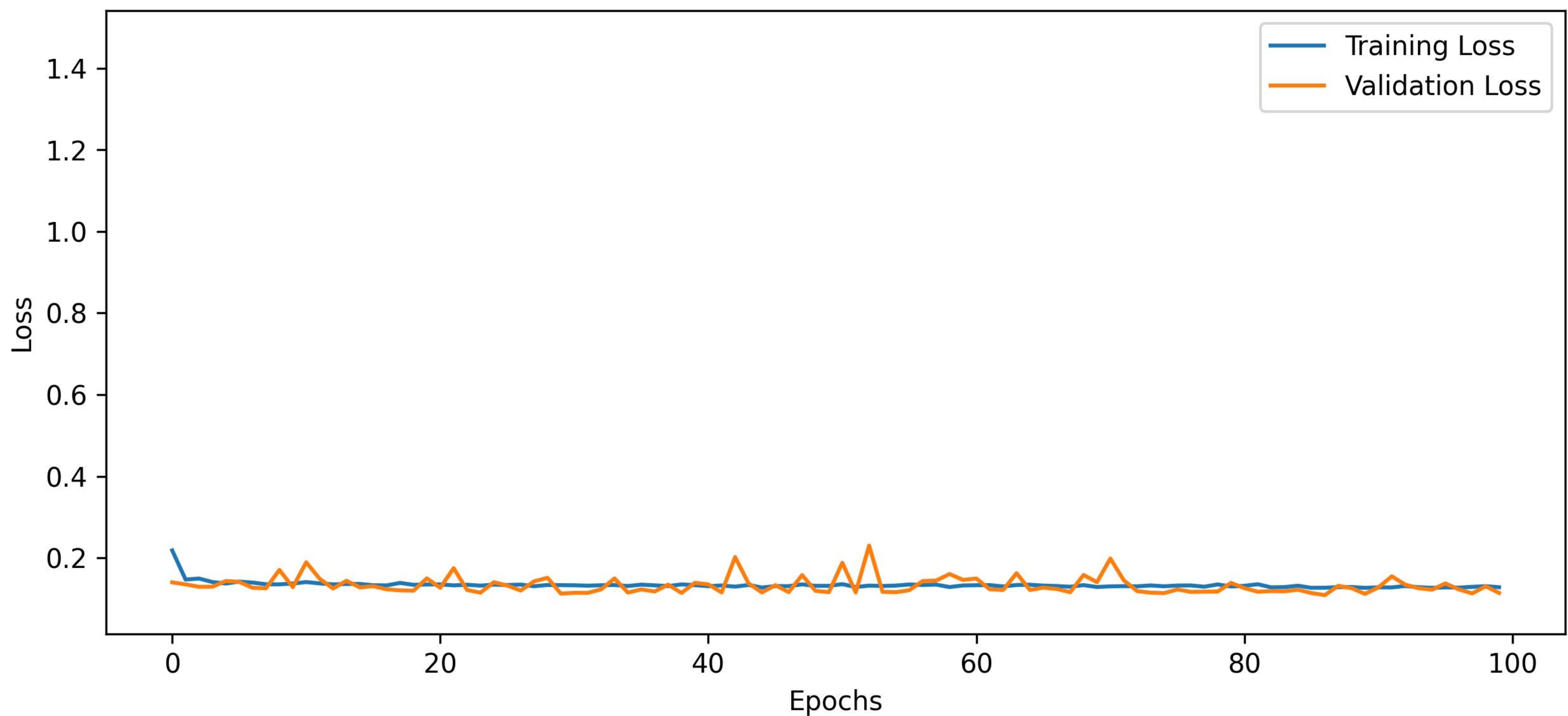
Dense
