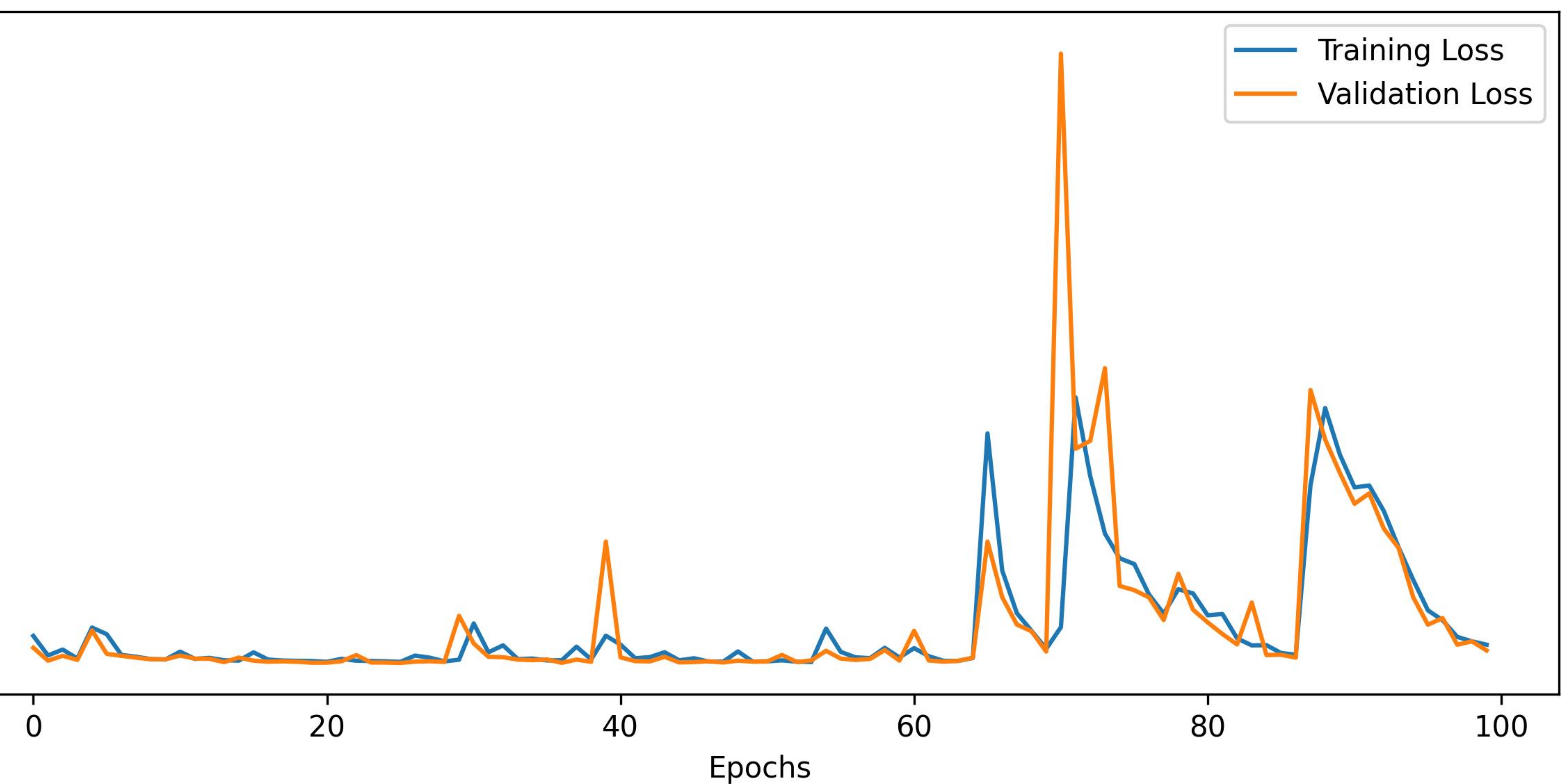
BLSTM
