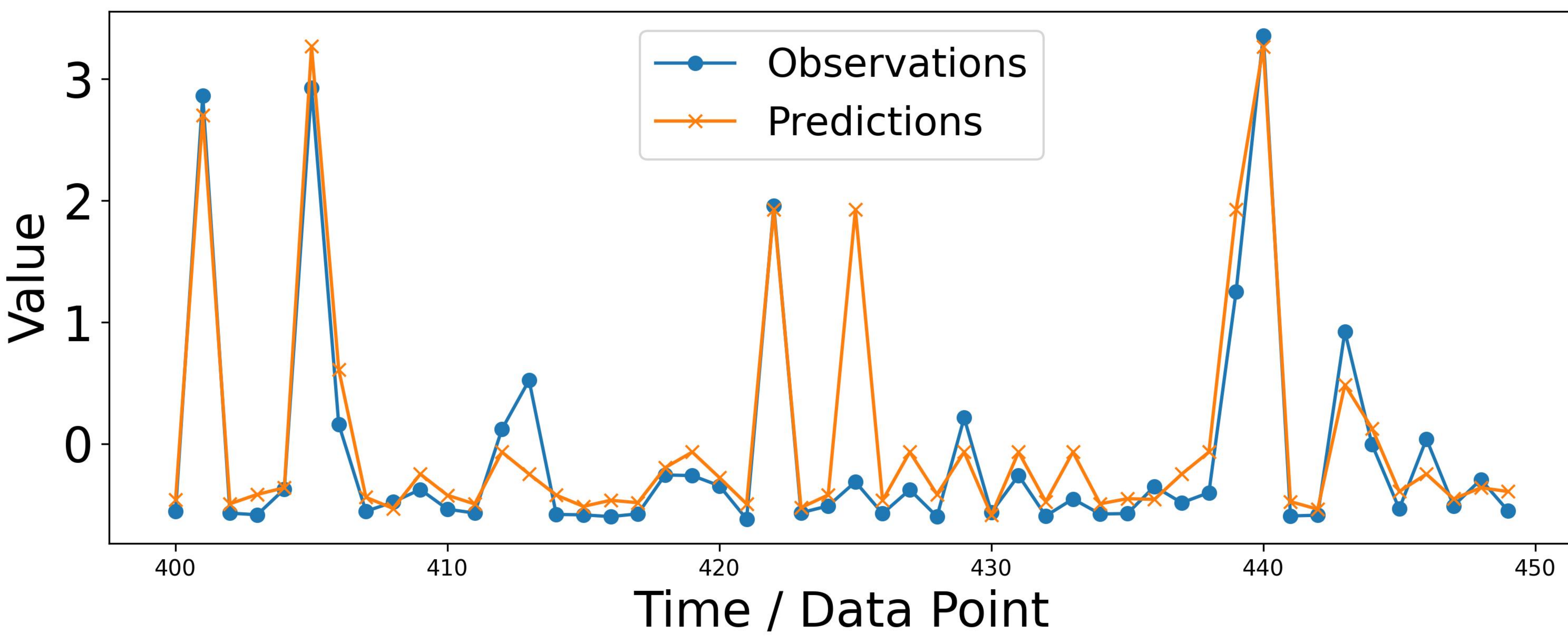
BLSTM
